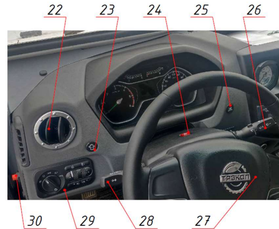
Рис. 5.9 Приборная панель
