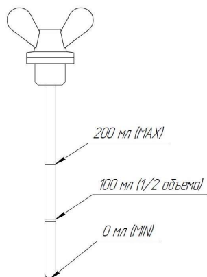
Рисунок 20.4. Указатель уровня антифриза
