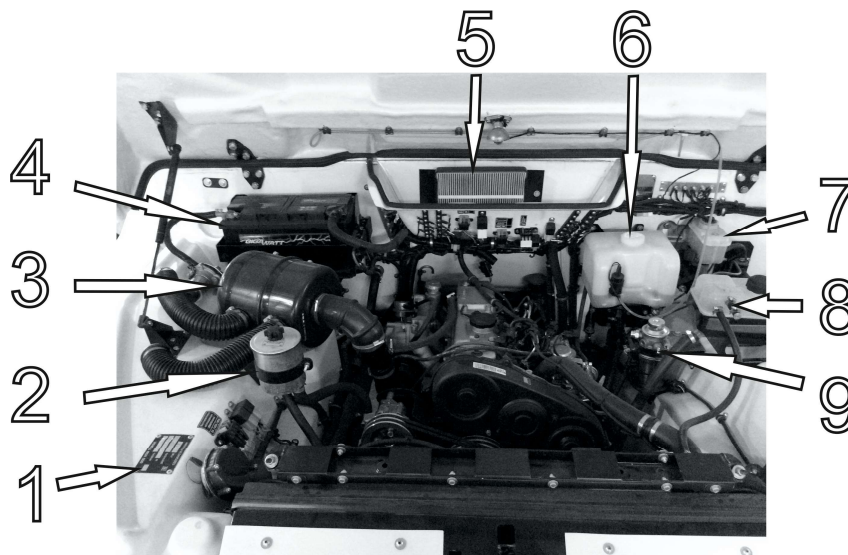
Рис. 4.1 Подкапотное пространство:
