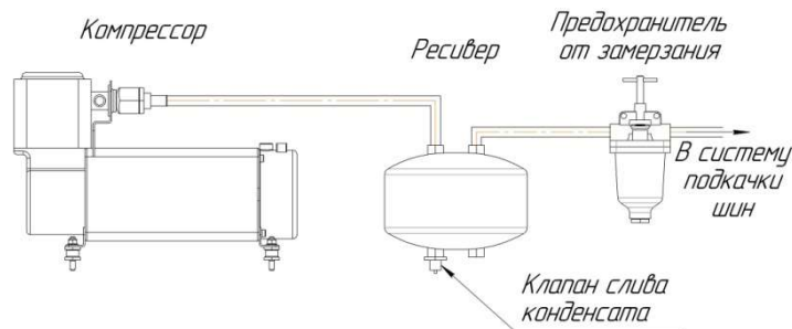
Рисунок 20.5. Схема системы предохранения СРДВШ от замерзания
