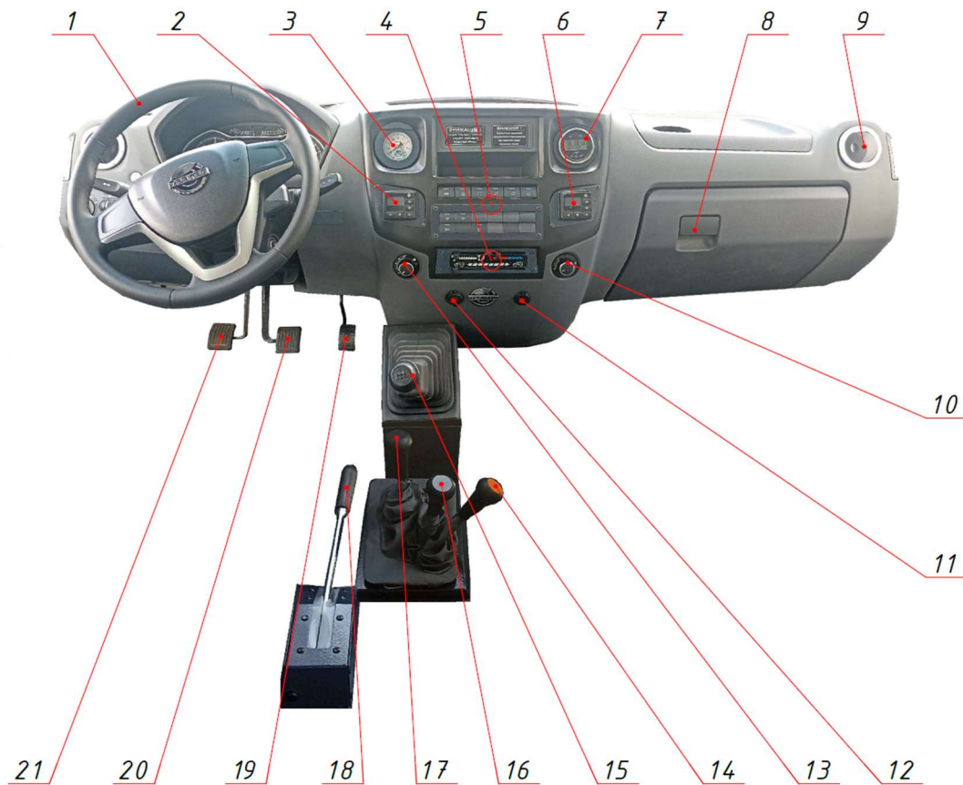
Рис. 5.4 Органы управления
