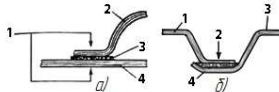
Рис. 6.37. Соединение слоистого пластика склеиванием:
