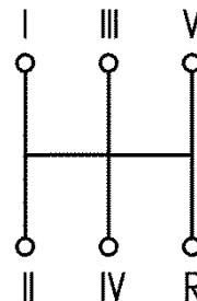
Рис. 6.1 Схема переключения коробки передач Hyundai DYMOS и ГАЗ А63R43
