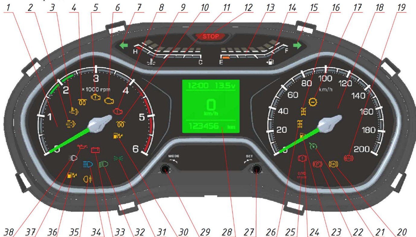
Рис. 5.2 Комбинация приборов
