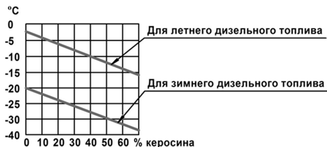
Рис. 20.16 Схема смешения дизельного топлива с керосином в зависимости от температуры окружающей среды.
