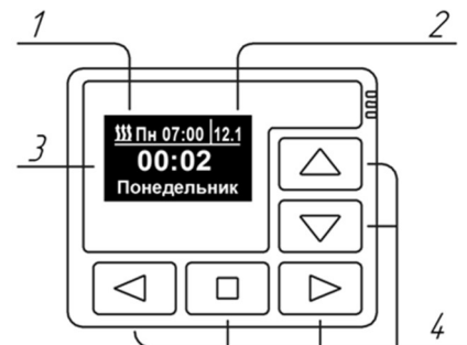
Рис. 20.18 Внешний вид пульта управления ПУ-40: 1 – активированный таймер запуска, 2 – напряжение питания, 3 – LED индикатор, 4 – кнопки управления.
