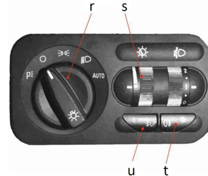
Рис. 5.13 Модуль управления светотехникой (вариант 1)
