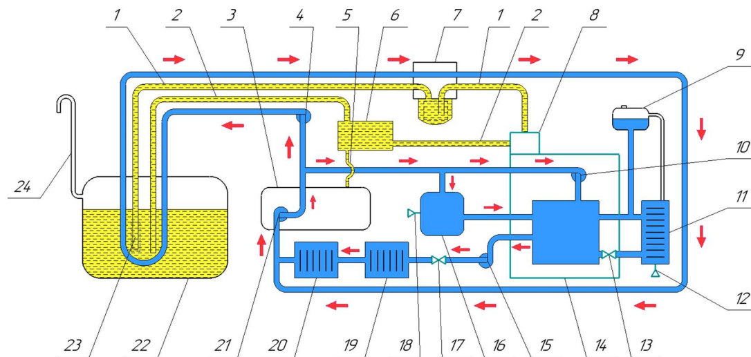
Рис. 20.20 Схема работы системы жидкостного подогрева топливной магистрали
