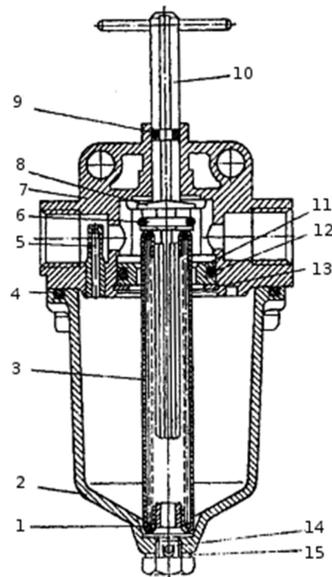
Рис. 20.3 Предохранитель от замерзания
