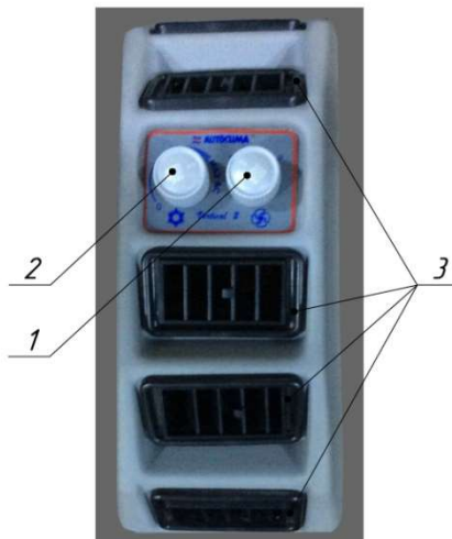
Рис.20.21 Блок кондиционера
