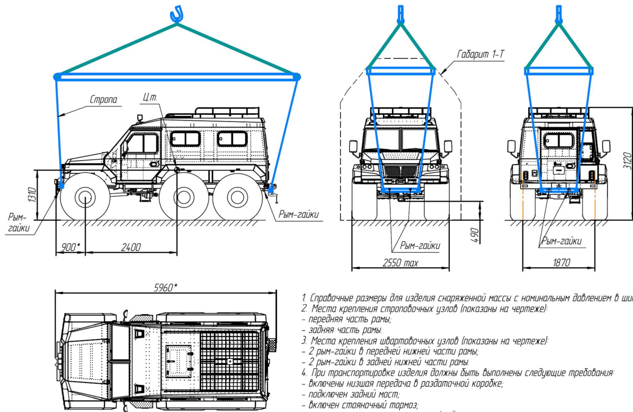
Рис. 15 Расположение строповочных и швартовочных узлов ВТС
