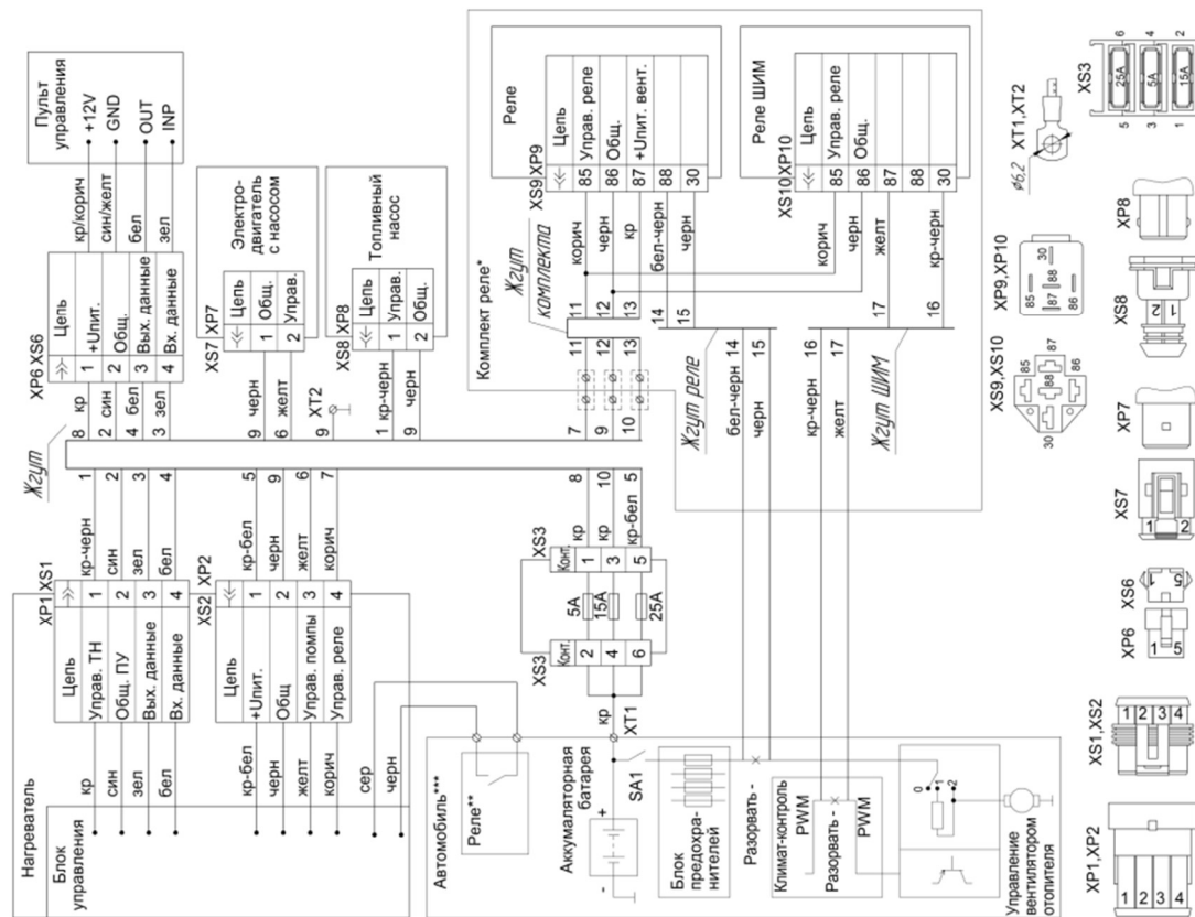
Рис. 20.14 Электрическая схема подключения подогревателя
