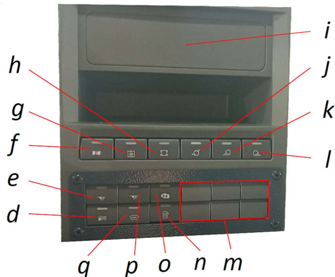
Рис. 5.6 Центральная панель
