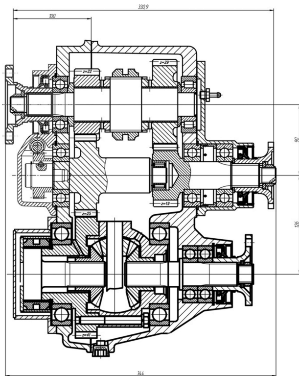
Рис.6.11 Коробка привода заднего ведущего моста с приводом водомётного движителя
