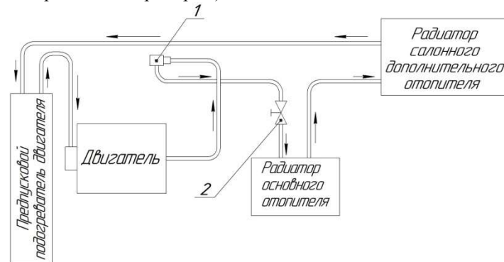
Рис. 6.29. Система отопления:
