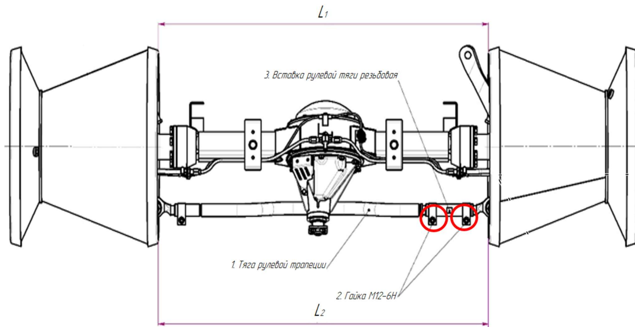
Рис. 6.16 – Регулировка схождения колёс.
