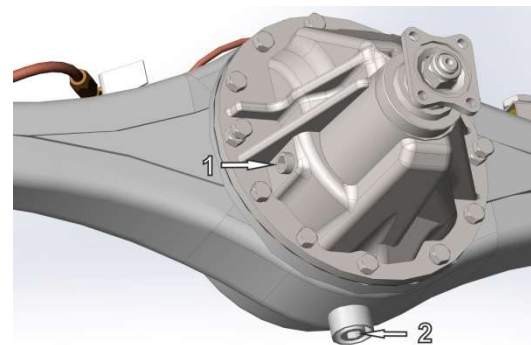
Рис. 9.5 Картер главной передачи ведущего моста: 1 - пробка заливного (контрольного) отверстия, 2 - пробка сливного отверстия
