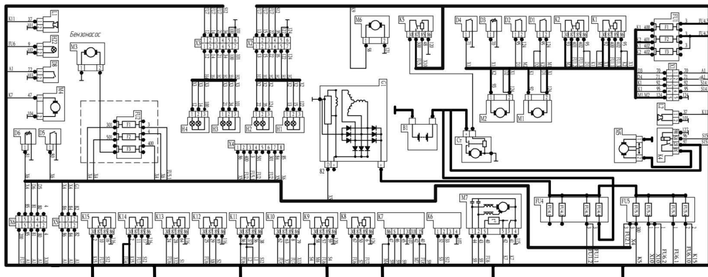
Рис 6.28 (Часть 1) Базовая электрическая схема ВТС.
