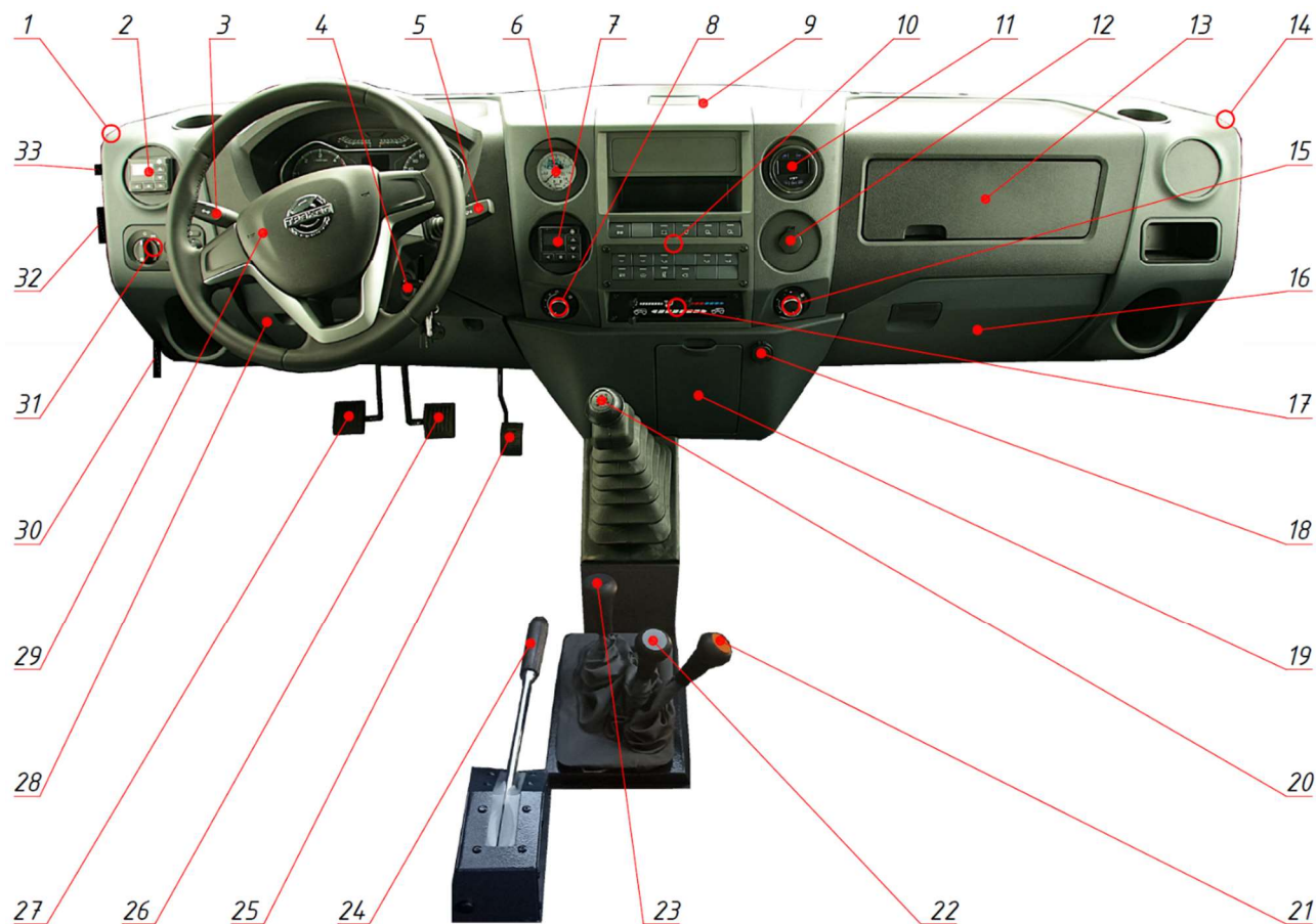
Рис. 5.5 Органы управления
