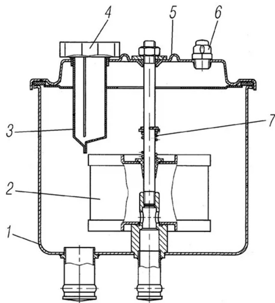
Рис. 6.15 Бачок усилителя рулевого управления:
