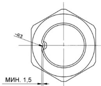
Рис. 6.21. Фиксация стопорной гайки
