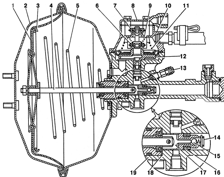
Рис. 6.26 Гидروвакуумный усилитель
