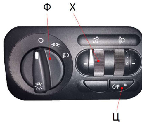
Рис. 5.14 Модуль управления светотехникой (вариант 1)
