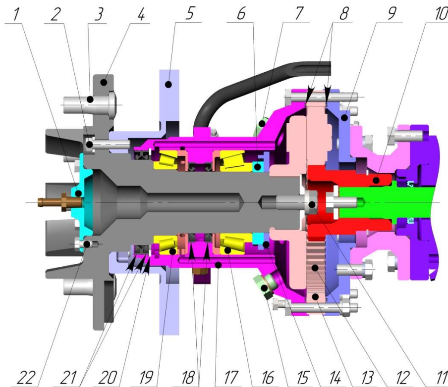
Рис. 6.12 Колесный редуктор
