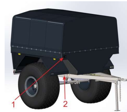
Рис. 2 Место обозначения заводского номера прицепа и расположение таблички заводских данных:
