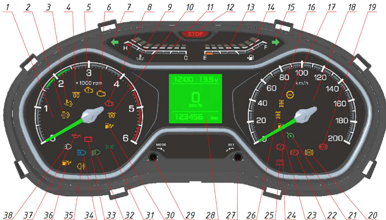
Рис. 5.2 Комбинация приборов
