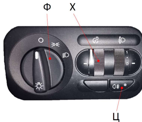
Рис. 5.12 Модуль управления светотехникой (вариант 1)
