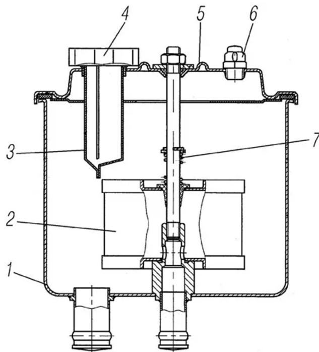
Рис. 6.18 Бачок усилителя рулевого управления: 1 – корпус; 2 – элемент фильтрующий; 3 – фильтр заливной; 4 – пробка; 5 – крышка; 6 – клапан предохранительный; 7 – пружина фильтра.
