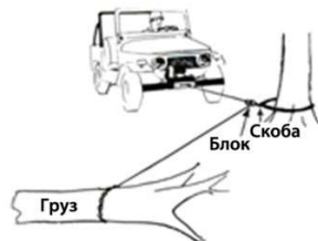
Рис. 19.9 Пример того, как с помощью блока можно менять направление тяги. Блок подсоединяется к древозащитной ленте с помощью соединительной скобы
