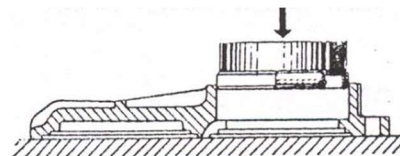
Рис.6.15 Запрессовка манжеты
