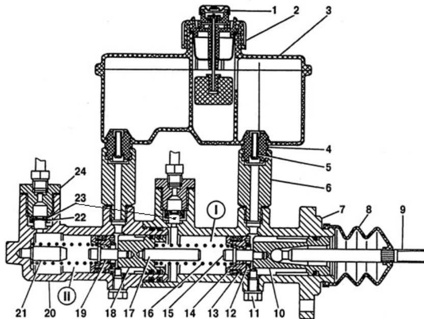
Рис.6.27 Главный тормозной цилиндр
