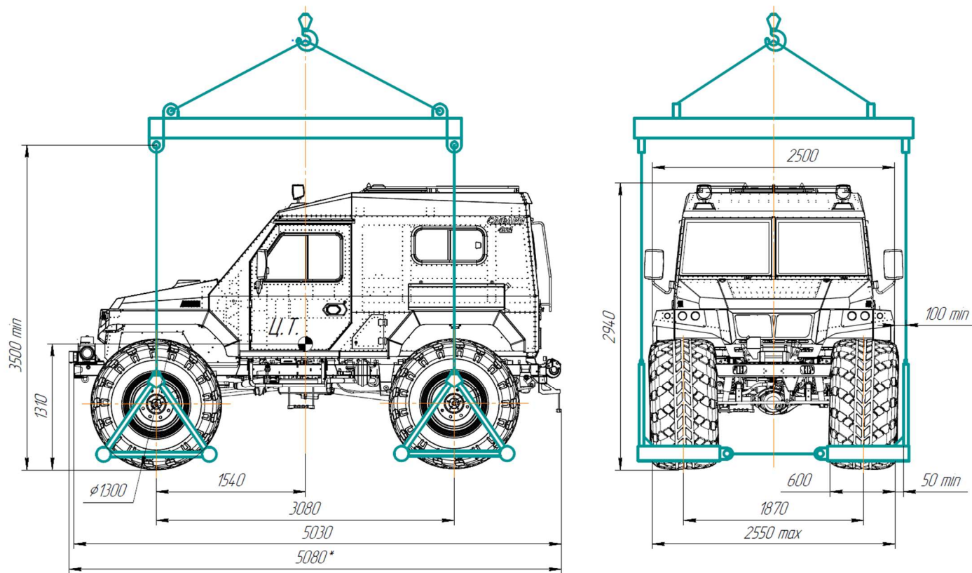
Рис. 14.2 Схема строповки ВТС
