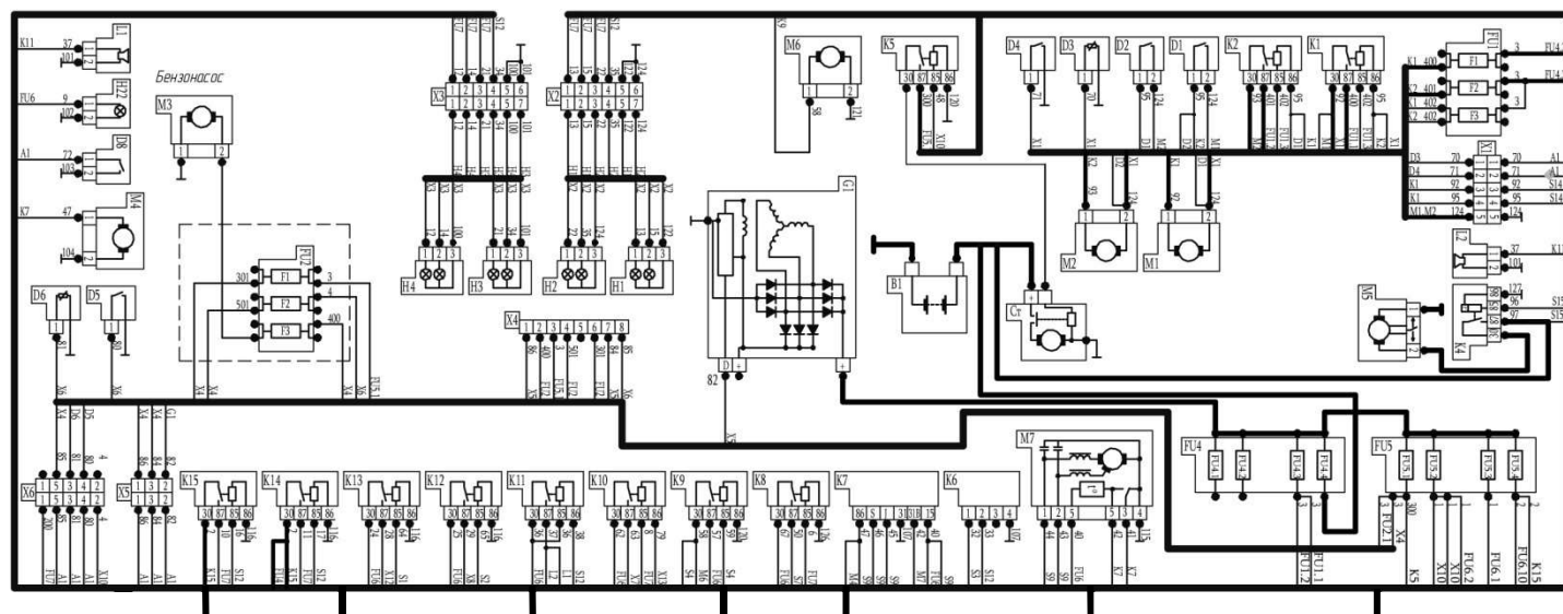
Рис 6.30 (Часть 1) Базовая электрическая схема ВТС
