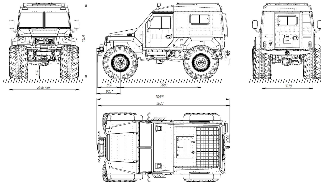
Рис. 5.1 Основные размеры ВТС ТРЭКОЛ САФАРИ
