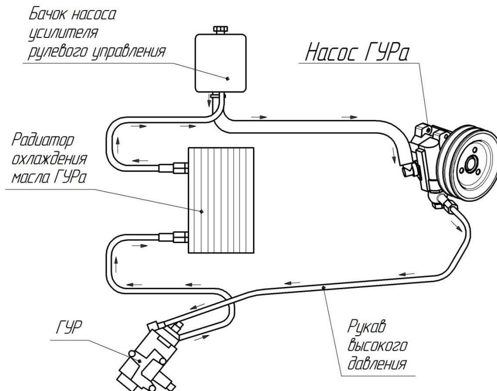
Рис. 6.17 Общая схема гидросистемы рулевого управления
