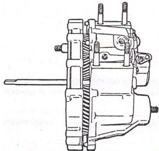
Рис.6.12 Разъединение переднего и заднего картеров
