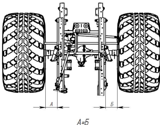
Рис. 6.19 Установка управляемых колес в положение прямолинейного движения.
