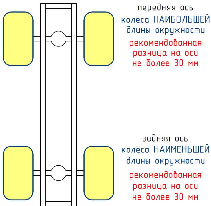
Рис. 10.1 Расстановка колёс
