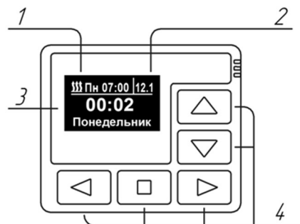
Рис. 19.18 Внешний вид пульта управления ПУ-40: 1 – активированный таймер запуска, 2 – напряжение питания, 3 – LED индикатор, 4 – кнопки управления.
