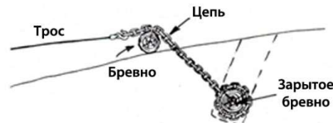
Рис. 19.13 Зарытое в землю бревно – отличный якорь. При необходимости вместо бревна можно использовать целый ряд предметов, например, металлическую балку, трубу или даже большую канистру.
