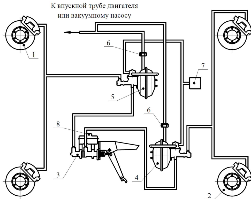
Рис. 6.26 Схема гидропривода тормозов:
