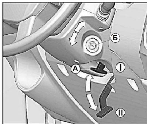
Рис. 5.6 Рычаг механизма фиксации рулевой колонки и замок выключателя приборов и стартера
