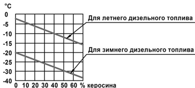
Рис. 19.16 Схема смешения дизельного топлива с керосином в зависимости от температуры окружающей среды.
