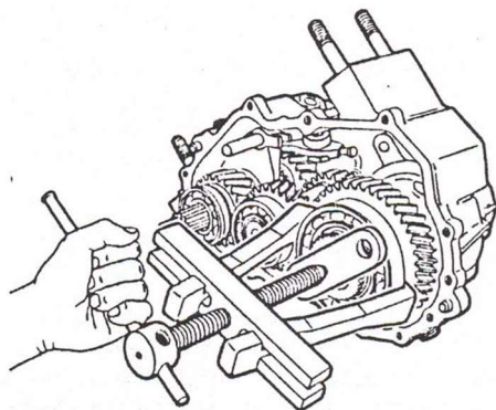
Рис.6.14 Спрессовка подшипника с шестерней дифференциала
