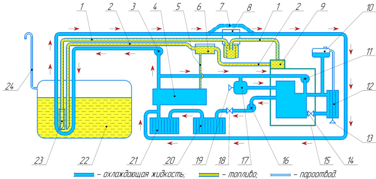
Рис. 19.20 Схема работы системы жидкостного подогрева топливной магистрали
