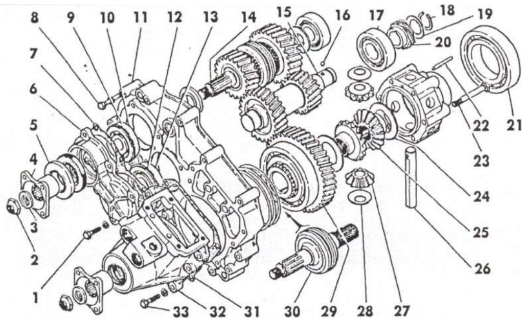
Рис.6.11 Детали переднего картера раздаточной коробки:
