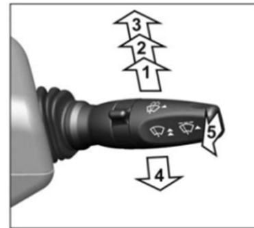
Рис. 5.8 Положения рычага переключателя стеклоочистителя и стеклоомывателя
