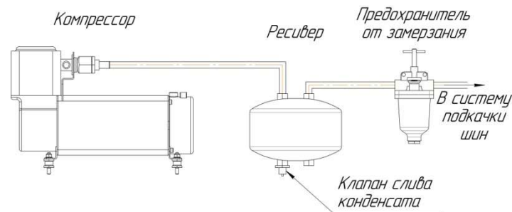
Рисунок 19.5. Схема системы предохранения СРДВШ от замерзания
