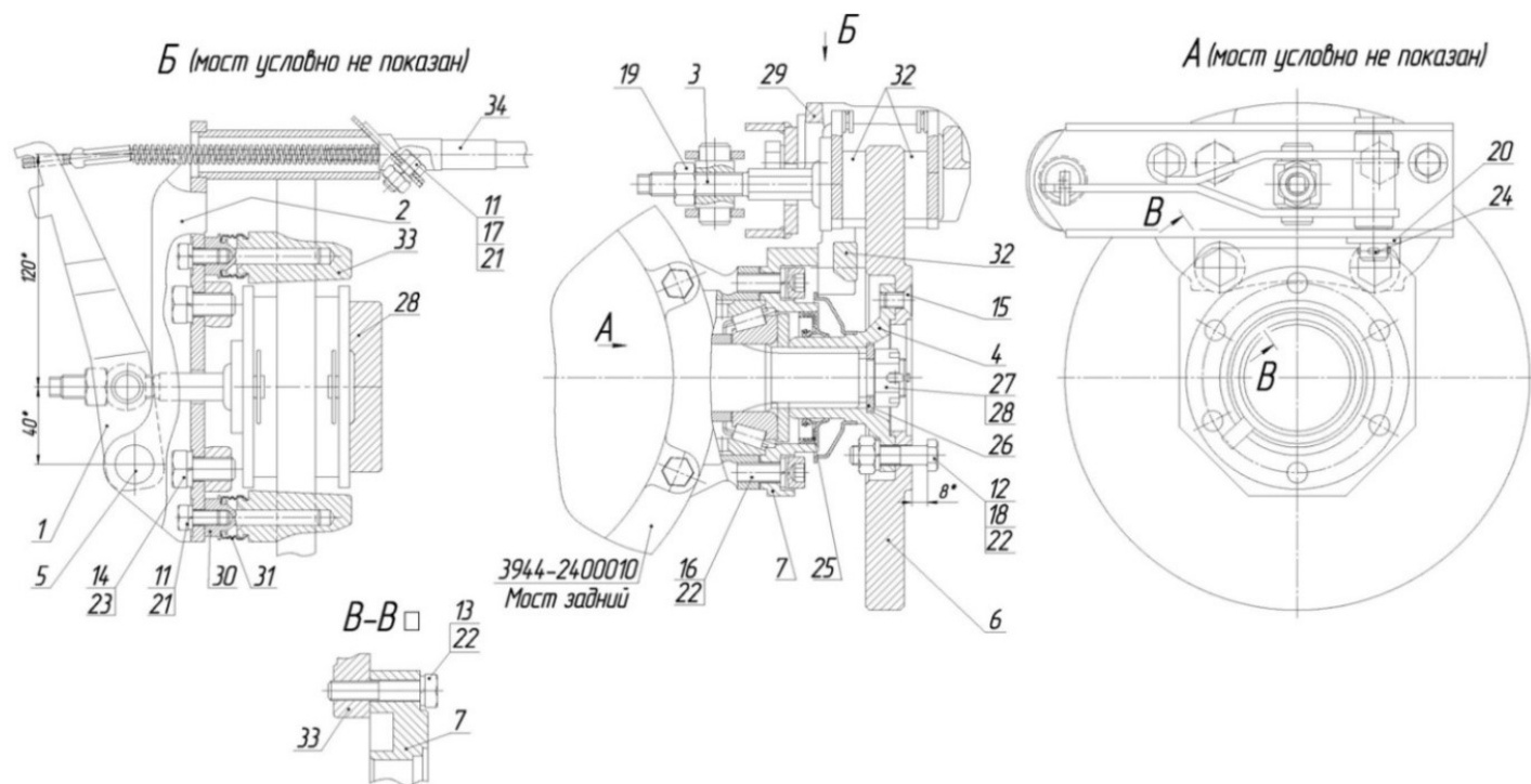
Рис. 6.29 Устройство стояночного тормоза
