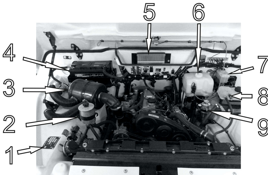
Рис. 4.1 Подкапотное пространство:
