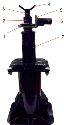
Рис. 12.1 Домкрат:
