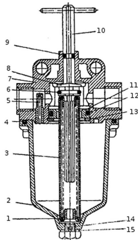
Рис. 19.3 Предохранитель от замерзания
