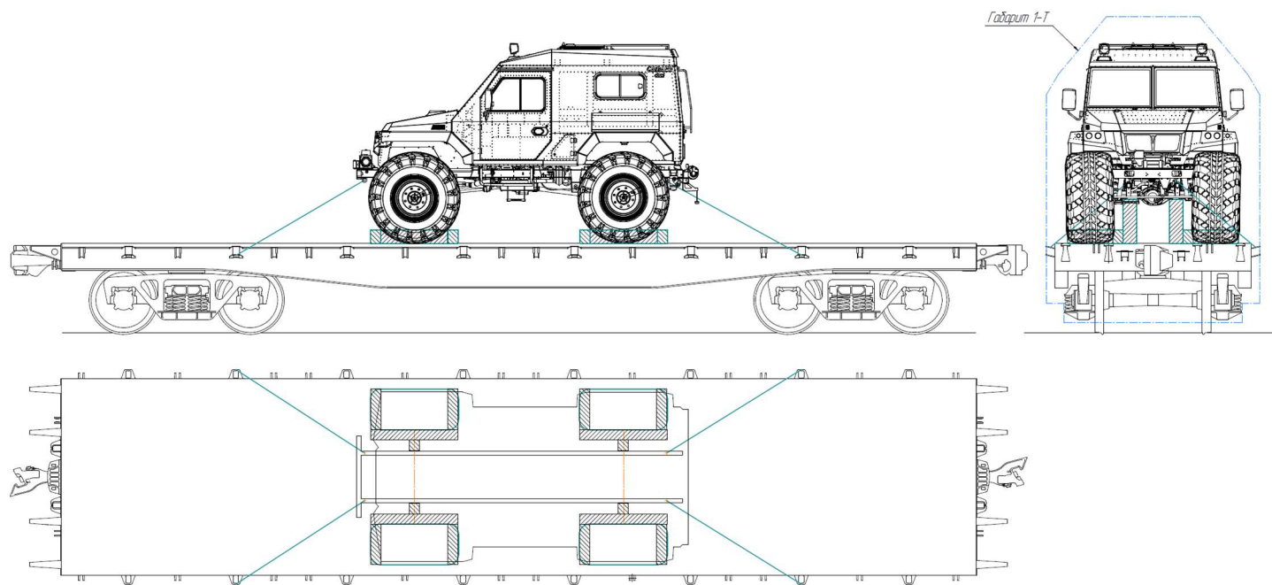
Рис. 14.1 Схема крепления ВТС на железнодорожной платформе
