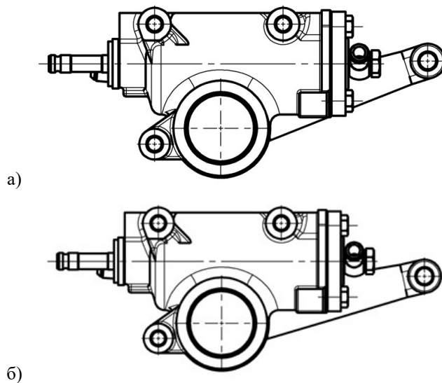
Рис. 6.23. Установка рулевой сошки
