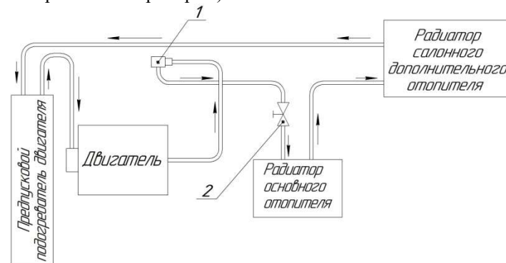
Рис. 6.31. Система отопления:
