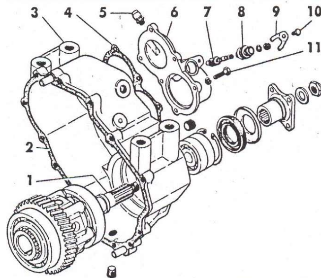
Рис.6.13 Детали заднего картера раздаточной коробки: 1 - вал привода заднего моста; 2 - прокладка; 3 - задний картер; 4 - прокладка; 5 - сапун; 6 - задняя крышка; 7 - ведомая шестерня привода спидометра; 8 - штуцер; 9 - стопор; 10 и 11 - болты
