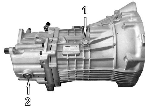
Рис. 9.2 Коробка передач ГАЗ А63R43 и ГАЗ А31R32:
