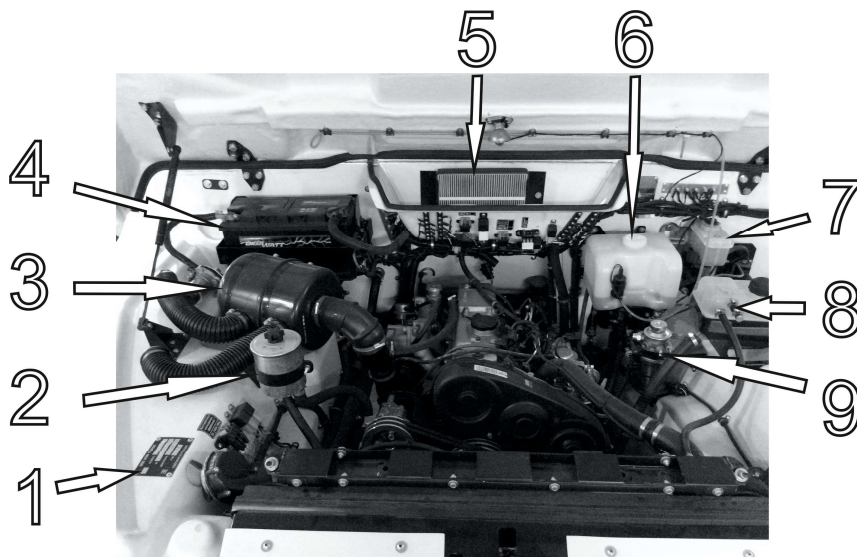
Рис. 4.1 Подкапотное пространство:
