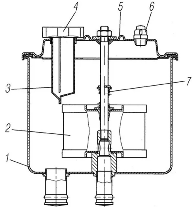
Рис. 6.18 Бачок усилителя рулевого управления: 1 – корпус; 2 - элемент фильтрующий; 3 – фильтр заливной; 4 – пробка; 5 - крышка; 6 – клапан предохранительный; 7 – пружина фильтра.
