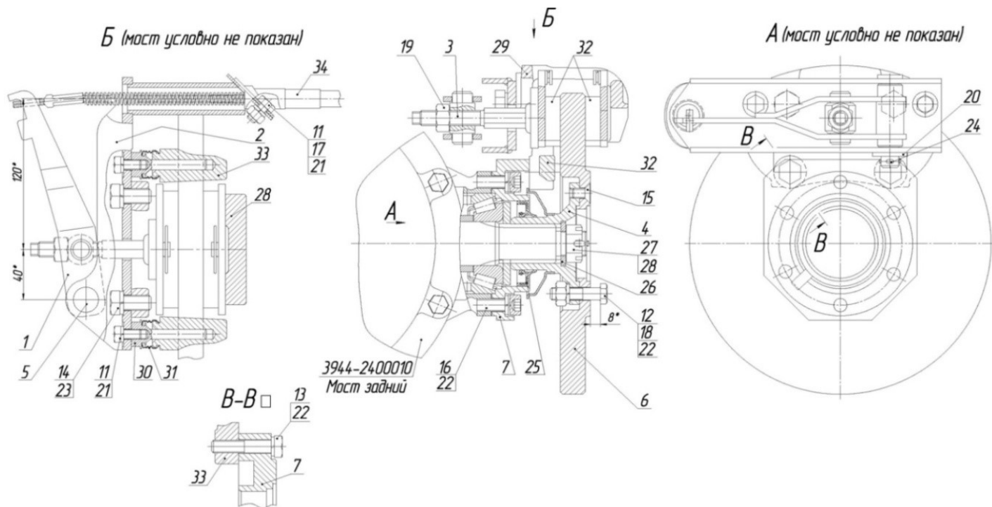
Рис. 6.27 Устройство стояночного тормоза
