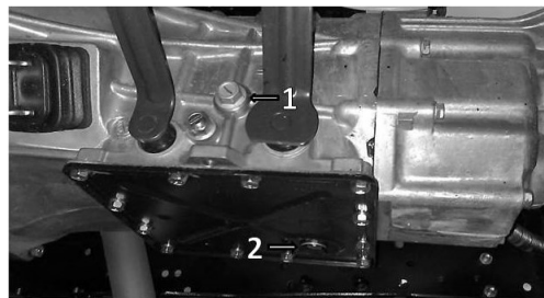
Рис. 9.1 Коробка передач HYUNDAI DYMOS M5ZR1: 1 - пробка заливного (контрольного) отверстия, 2 - пробка сливного отверстия.
