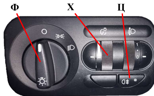
Рис. 5.12 Модуль управления светотехникой (вариант 1)
