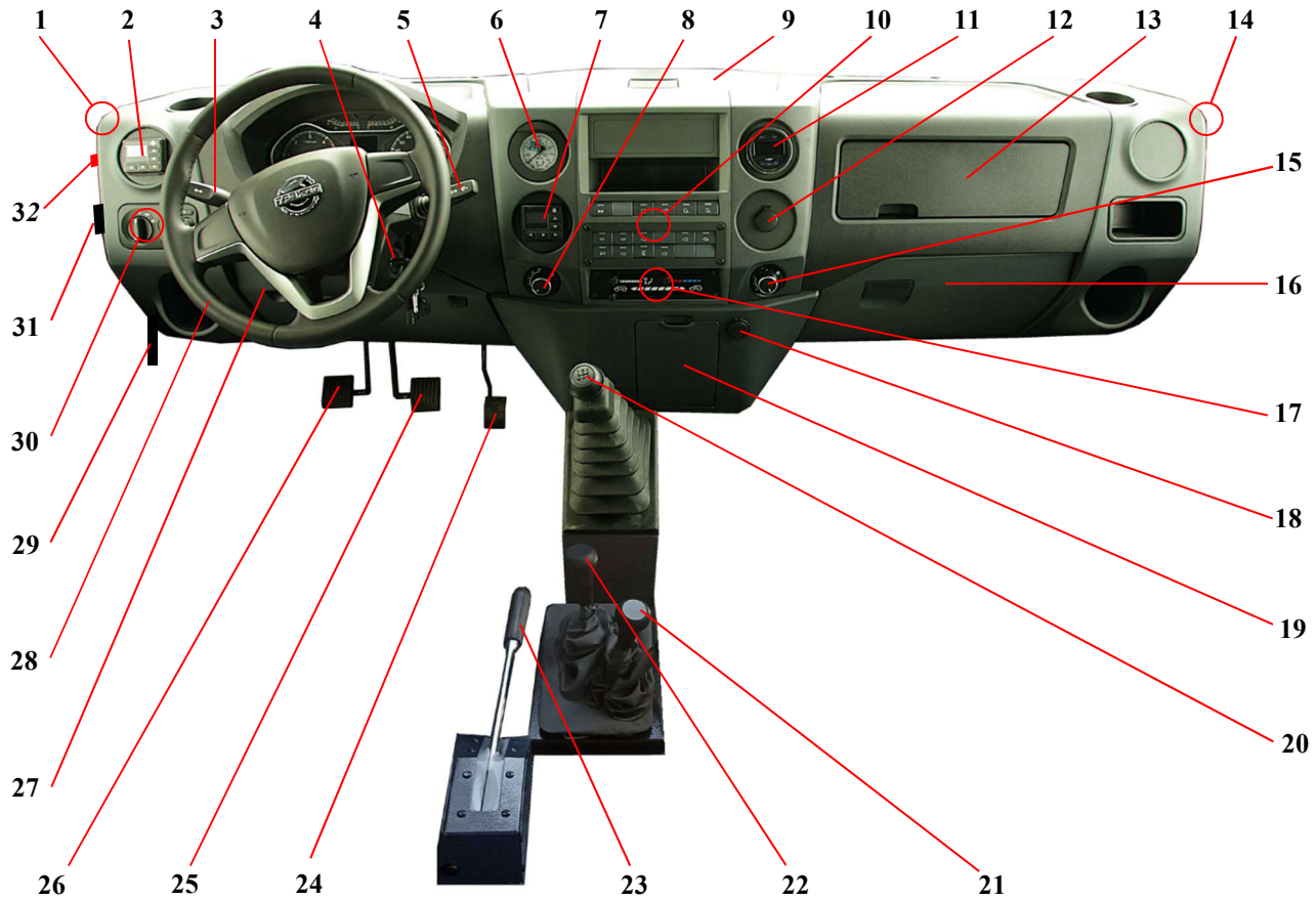
Рис. Ошибка! Текст указанного стиля в документе отсутствует..1 Органы управления
