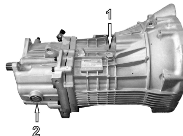
Рис. 9.2 Коробка передач ГАЗ А63R43 и ГАЗ А31R32: 1 - пробка заливного (контрольного) отверстия, 2 - пробка сливного отверстия.
