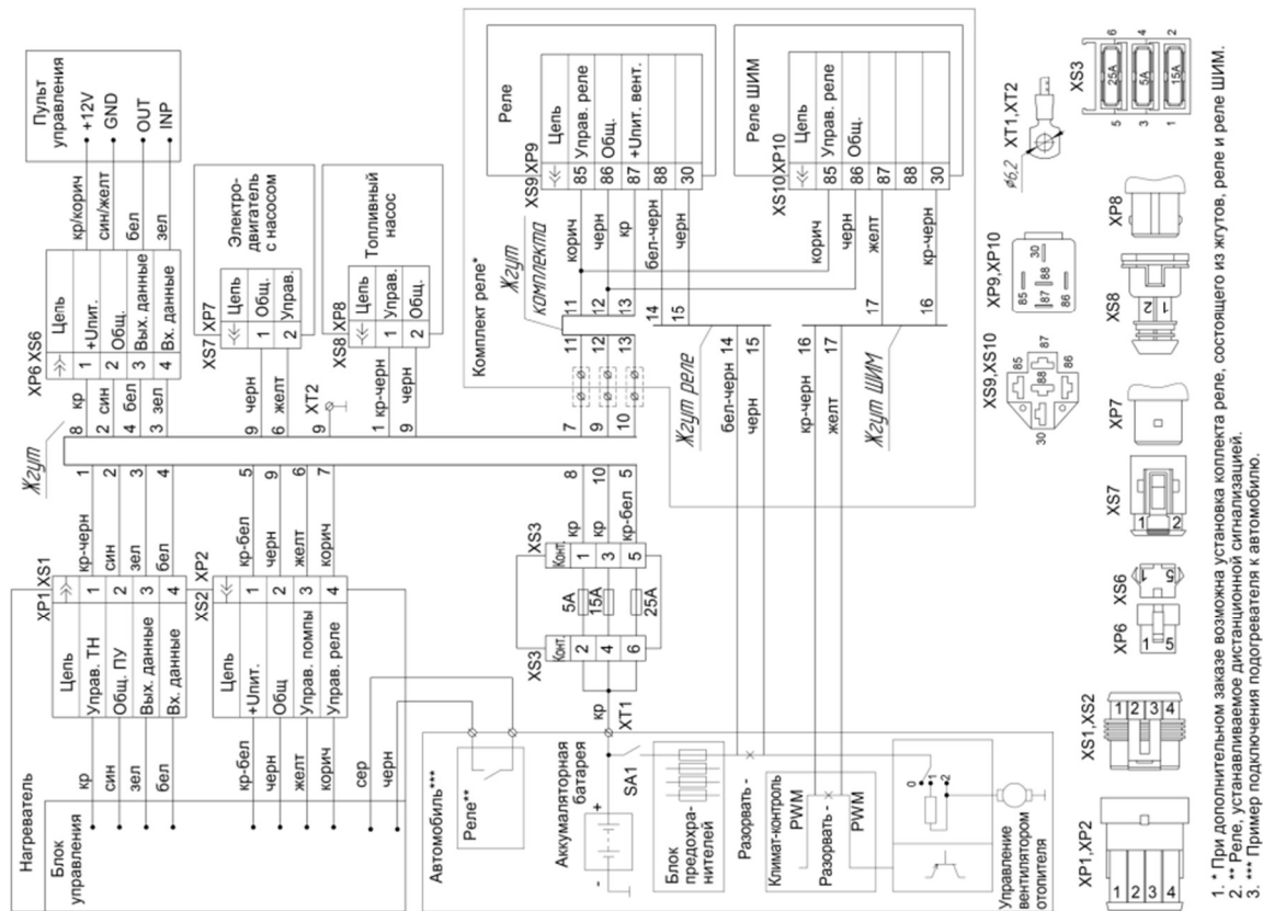
Рис. 19.15 Электрическая схема подключения подогревателя
