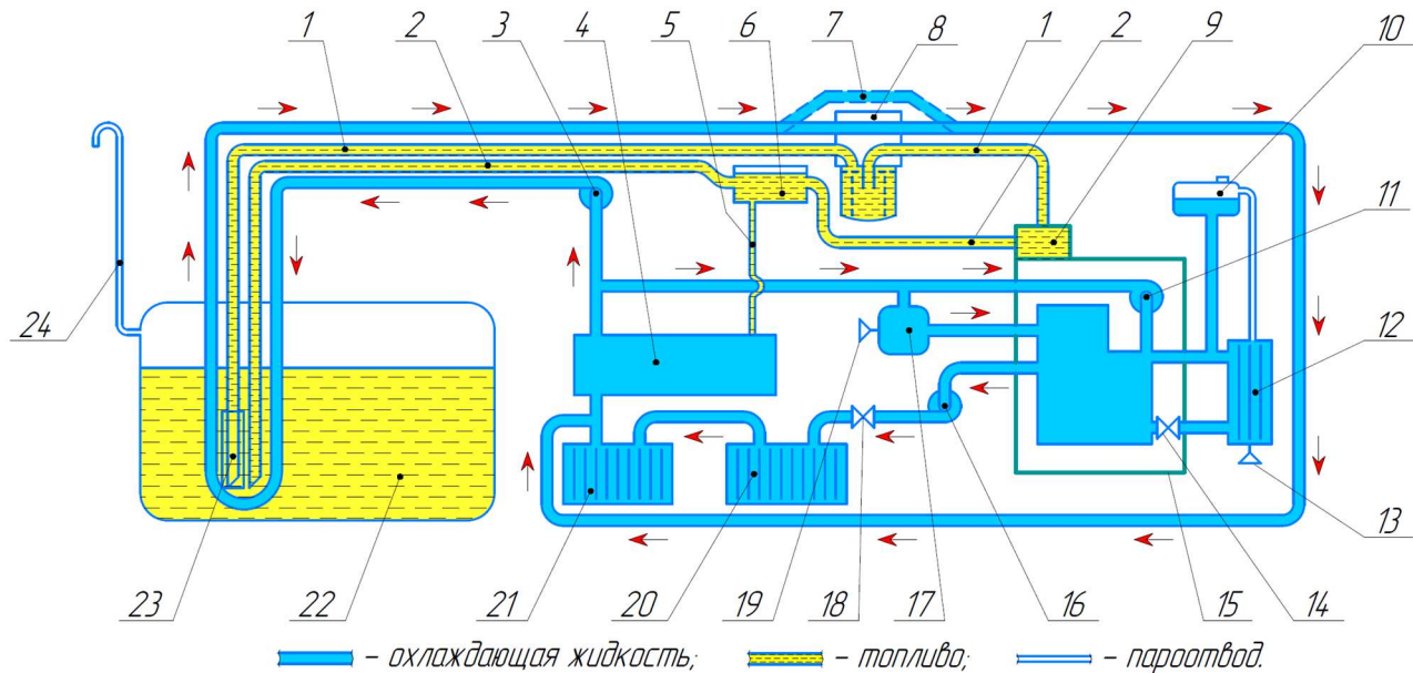
Рис. 19.20 Схема работы системы жидкостного подогрева топливной магистрали
