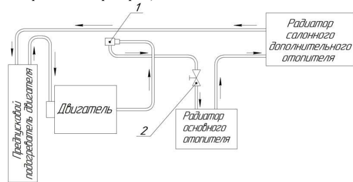
Рис. 6.28. Система отопления:
