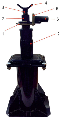
Рис. 12.1 Домкрат:
