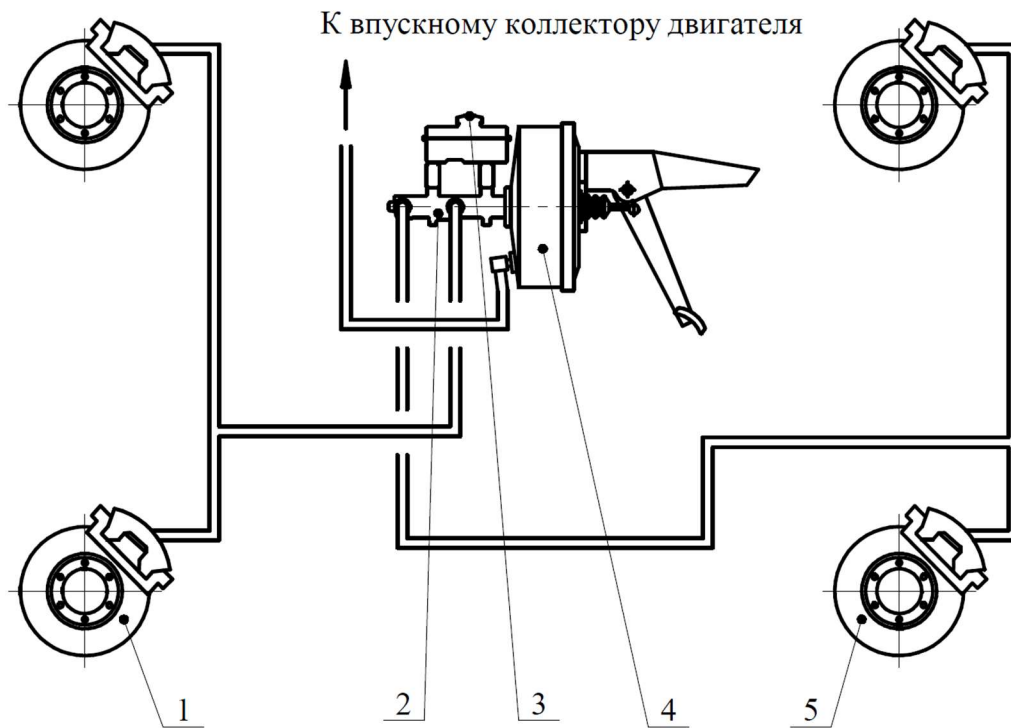
Рис. 6.26 Схема гидропривода тормозов:
