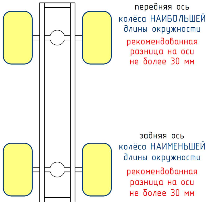
Рис. 10.1 Расстановка колёс
