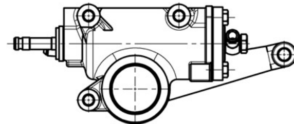
Рис. 6.23. Установка рулевой сошки
