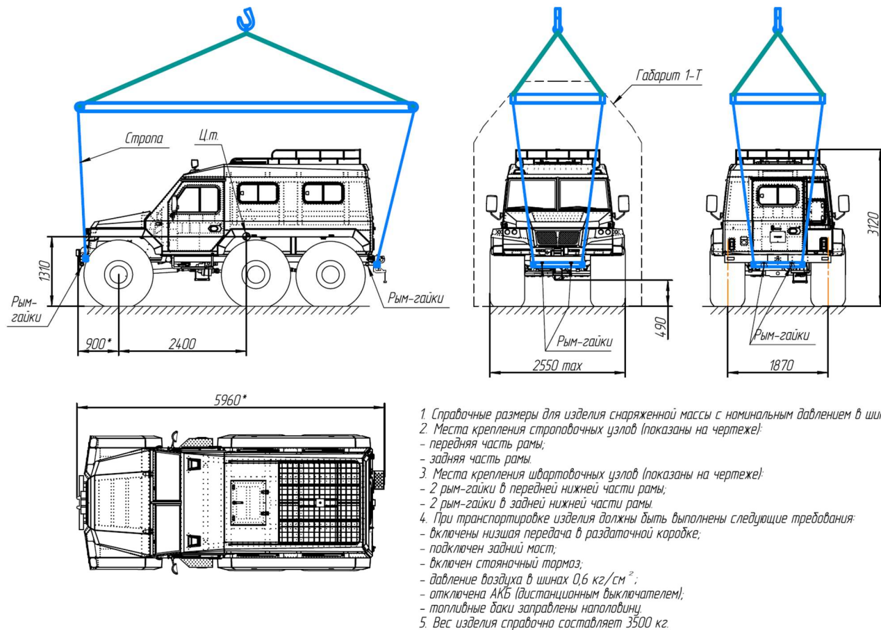
Рис. 15 Расположение строповочных и швартовочных узлов ВТС
