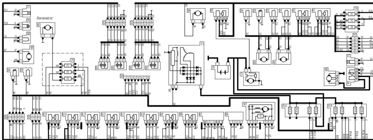
Рис 6.34 (Часть 1) Базовая электрическая схема ВТС
