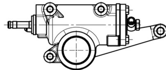
Рис. 6.18. Установка рулевой сошки
