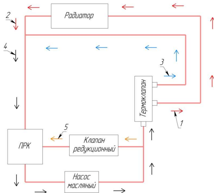
Рис. 6.4 Общая схема системы охлаждения ПРК
