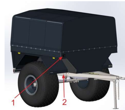
Рис. 2 Место обозначения заводского номера прицепа и расположение таблички заводских данных:
