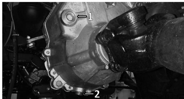
Рис. 9.3 Раздаточная коробка:
