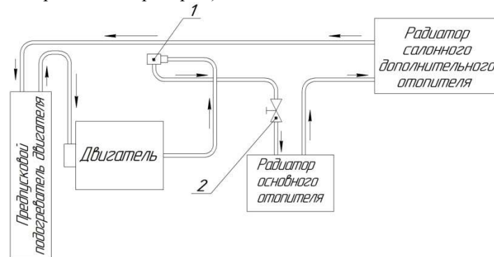
Рис. 6.29. Система отопления:
