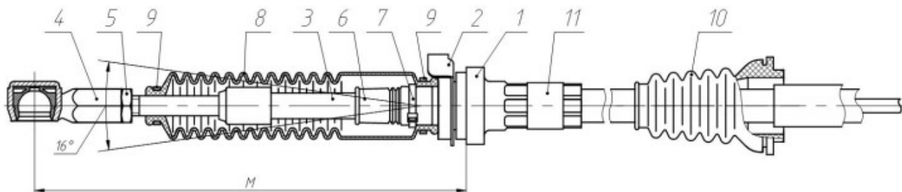
Рис. 6.3 Состав троса
