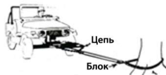
Рис. 20.7 В основном то же, что на рис. 20.6. Цепь с распределителем помогает равномерно распределить нагрузку по составным частям автомобиля
