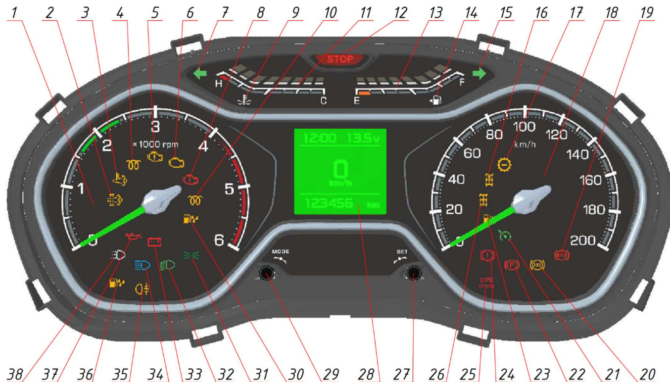
Рис. 5.3 Комбинация приборов
