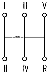
Рис. 6.1 Схема переключения коробок передач ГАЗ А63R43, Hyundai DYMOS и ГАЗ А31R32
