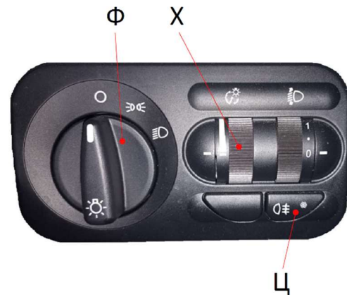
Рис. 5.14 Модуль управления светотехникой (вариант 1)
