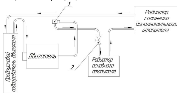
Рис. 6.35. Система отопления:
