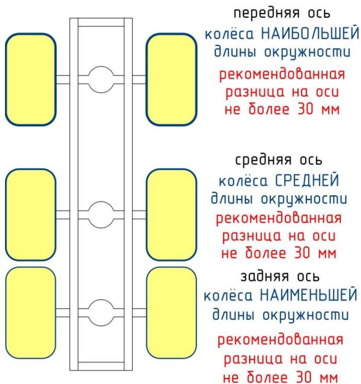
Рис. 10.1 Расстановка колёс
