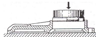
Рис.6.18 Запрессовка манжеты
