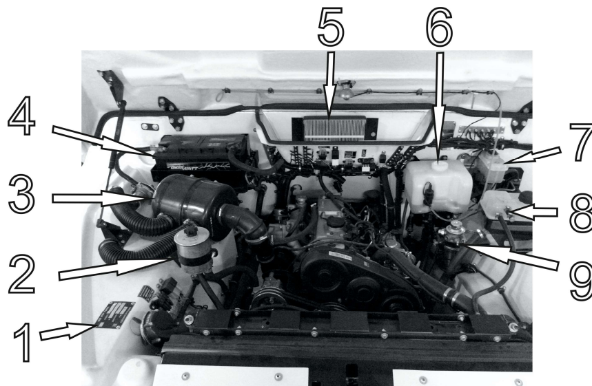
Рис. 4.1 Подкапотное пространство:
