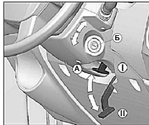
Рис. 5.7 Рычаг механизма фиксации рулевой колонки и замок выключателя приборов и стартера
