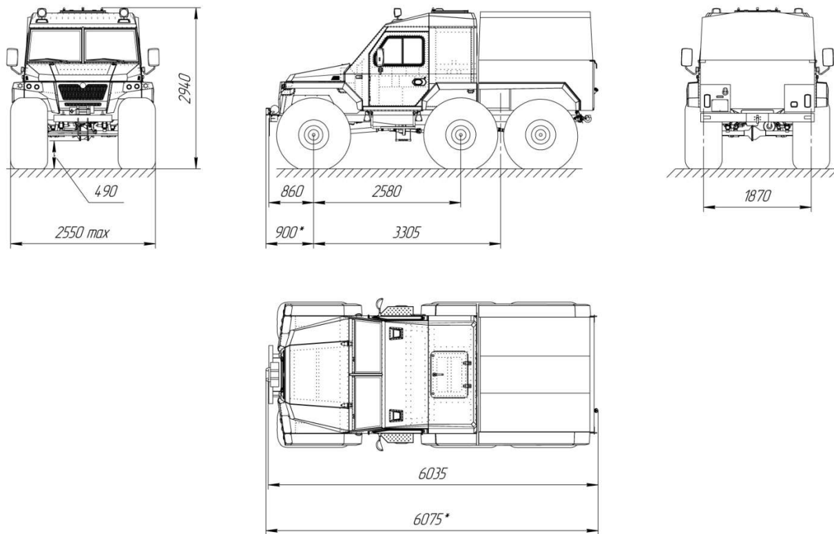
Рис. 5.2 Основные размеры ВТС ТРЭКОЛ ВЕГА Пикап
