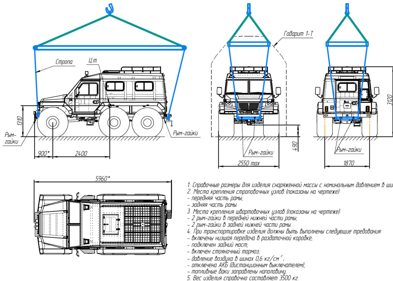
Рис. 15 Схема расположения строповочных и швартовочных узлов ВТС
