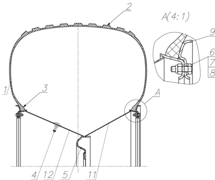
Рис. 10.3 Шина 1300х600-533 ТРЭКОЛ с колесом в сборе
