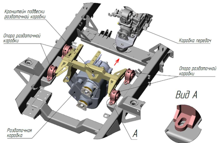
Рис. 6.19 Установка опор кронштейна подвески раздаточной коробки
