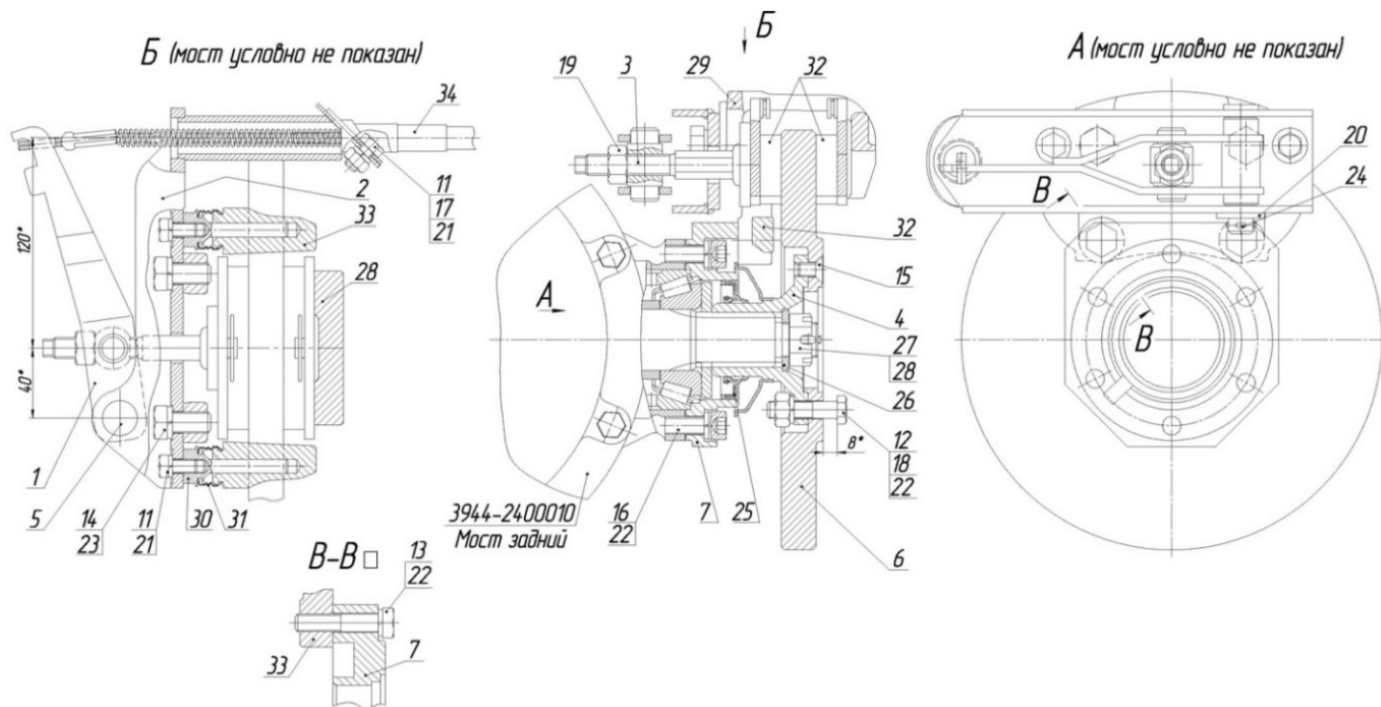
Рис. 6.33 Устройство стояночного тормоза
