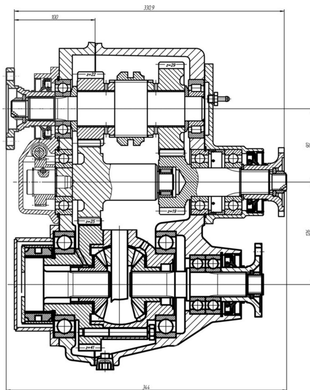
Рис.6.11 Коробка привода заднего ведущего моста с приводом водометного движителя
