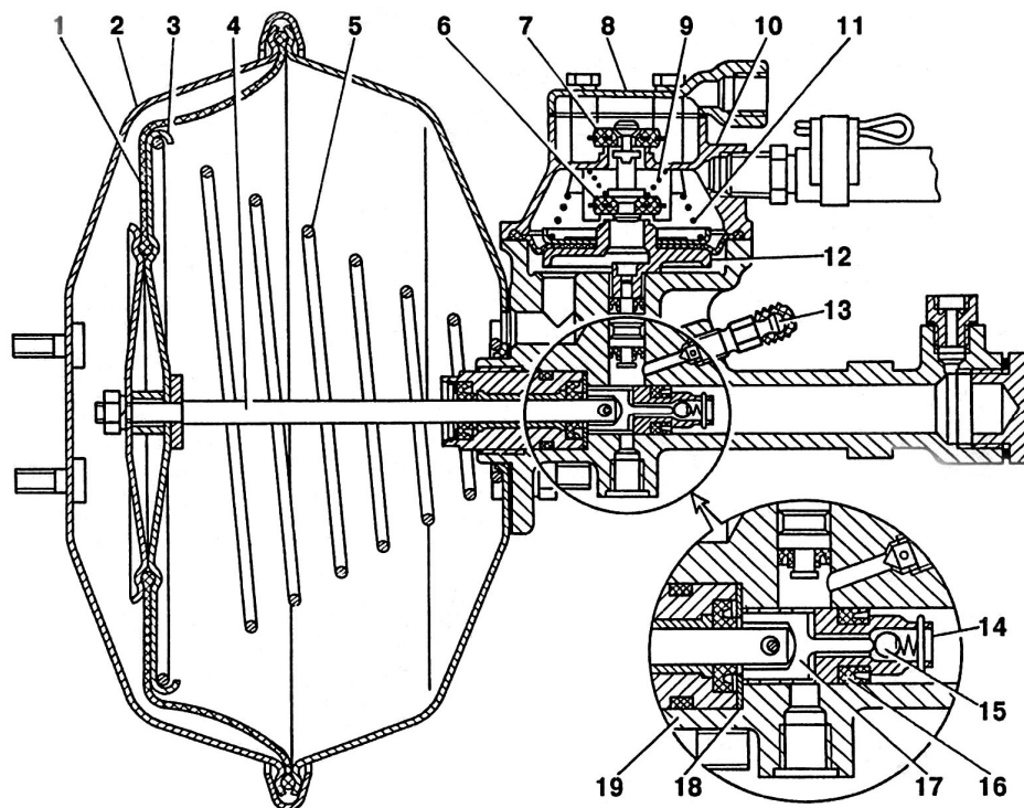
Рис. 6.32 Гидروвакуумный усилитель
