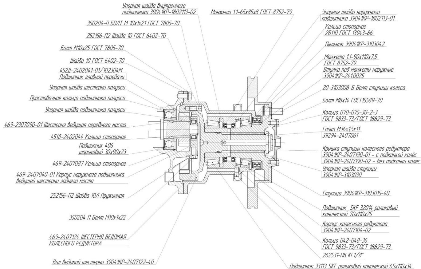
Рис. 6.20 Колесный редуктор ТРЭКОЛ
