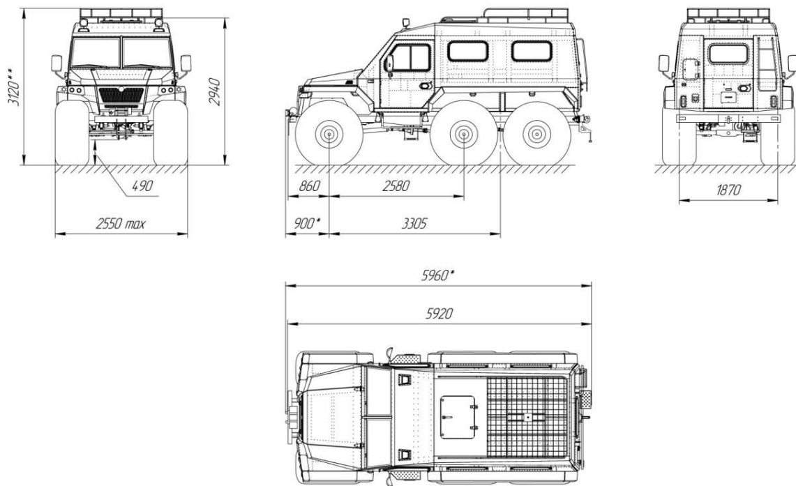
Рис. 5.1 Основные размеры ВТС ТРЭКОЛ ВЕГА
