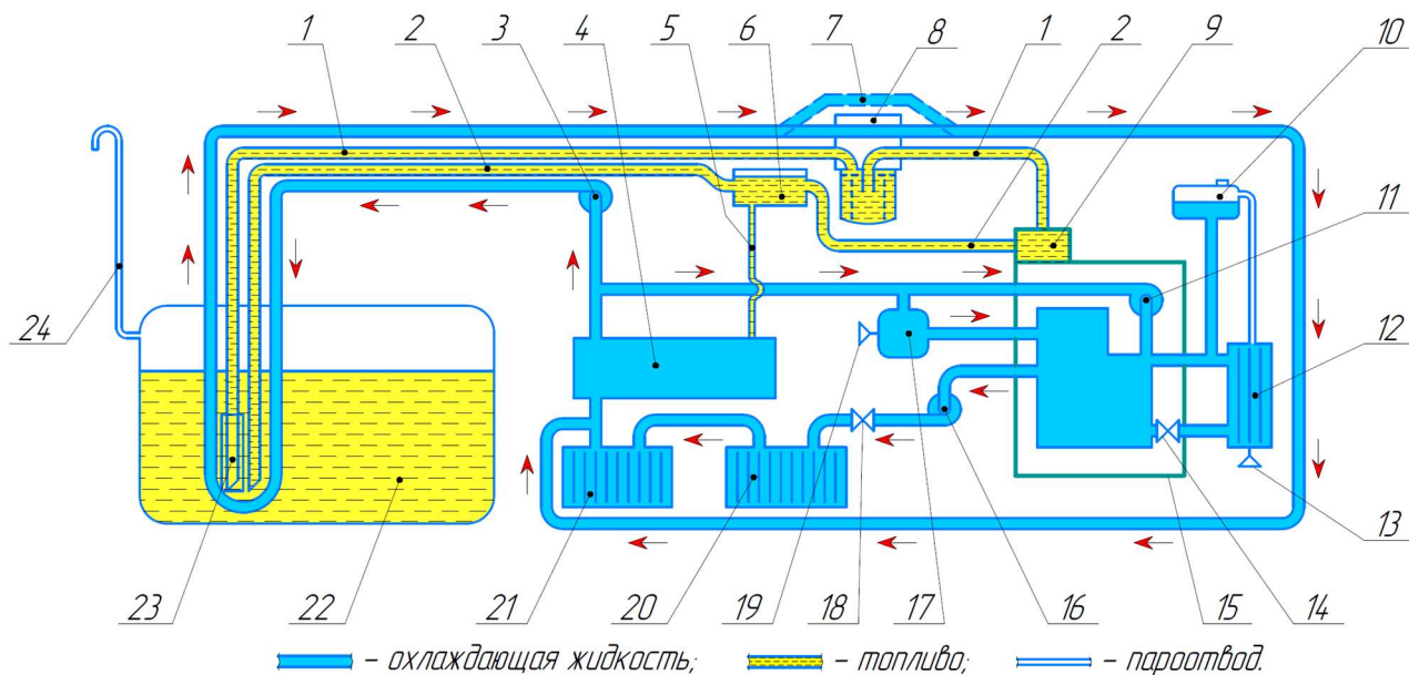
Рис. 20.19 Схема работы системы жидкостного подогрева топливной магистрали
