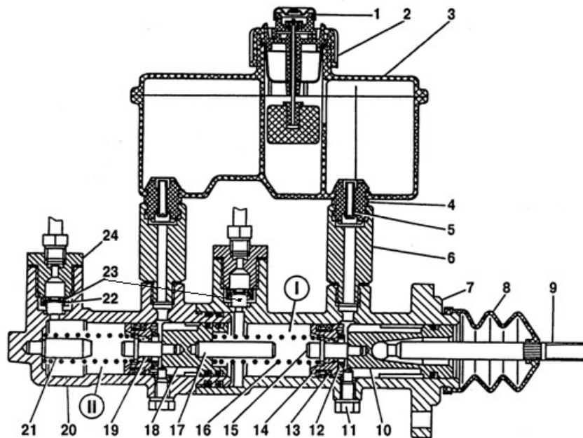
Рис.6.31 Главный тормозной цилиндр
