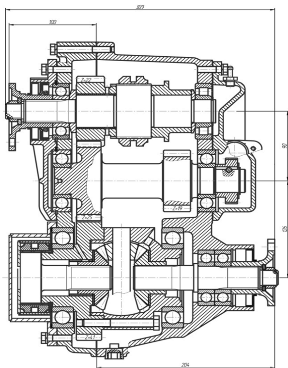
Рис.6.10 Коробка привода заднего ведущего моста
