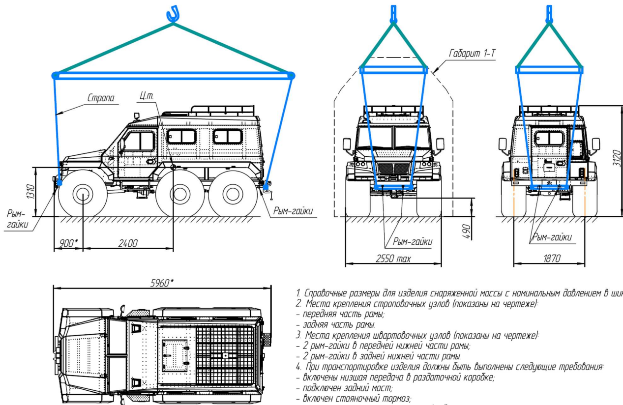
Рис. 15 Схема расположения строповочных и швартовочных узлов ВТС
