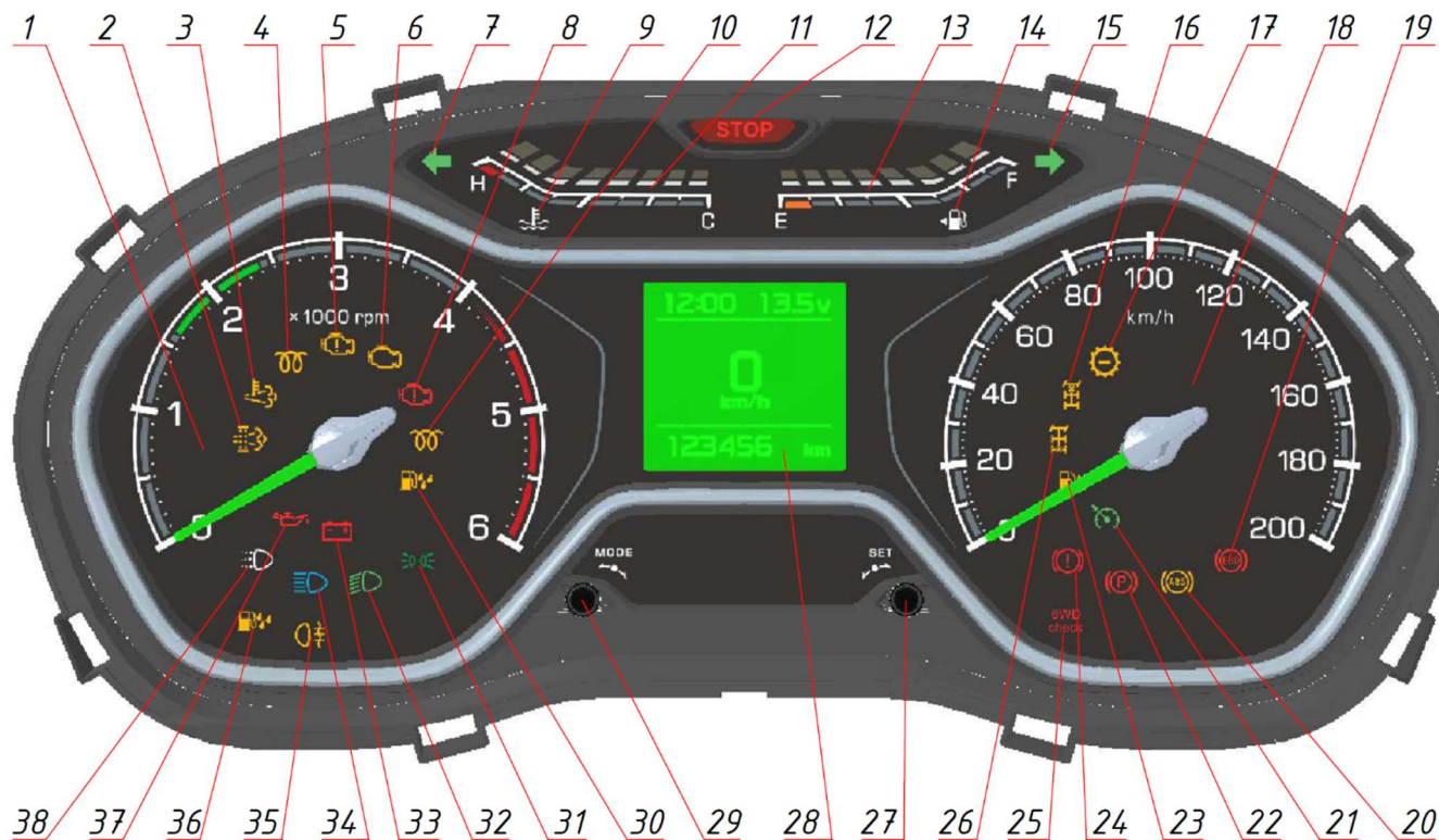
Рис. 5.3 Комбинация приборов
