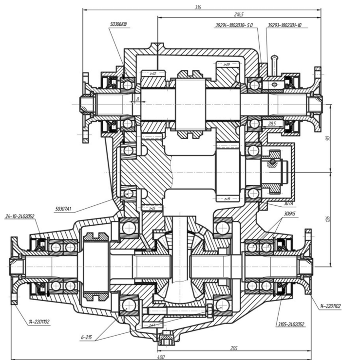
Рис.6.9 Коробка раздаточная (передняя)
