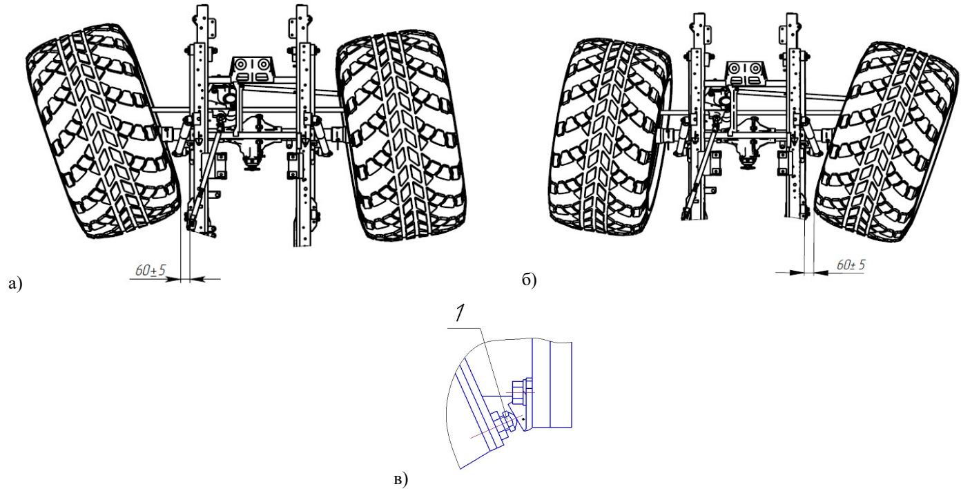
Рис. 6.25. Регулировка углов поворота колес. а) При повороте влево; б) При повороте вправо; в) Упор-ограничитель.
