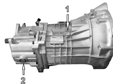
Рис. 9.2 Коробка передач ГАЗ А63R43 и ГАЗ А31R32:
