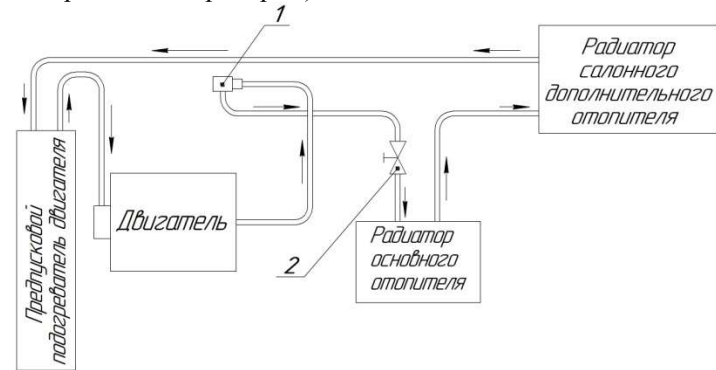
Рис. 6.34. Система отопления:
