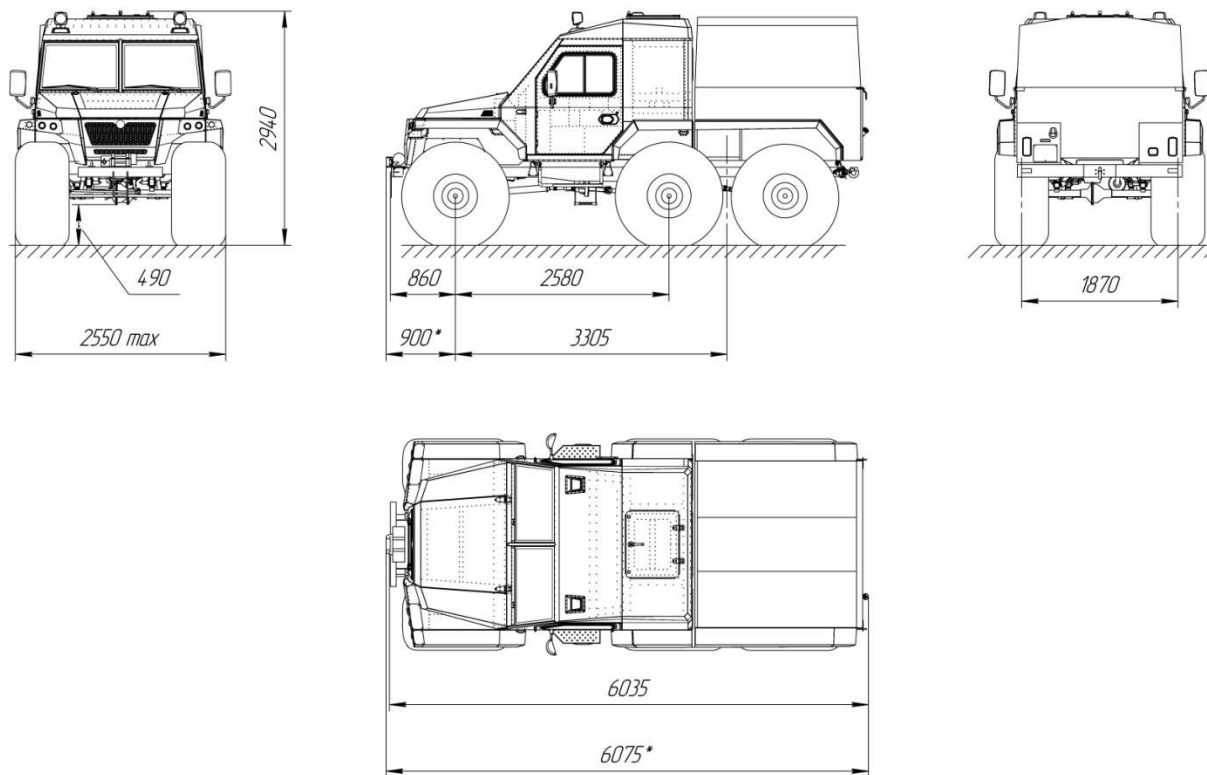
Рис. 5.2 Основные размеры ВТС ТРЭКОЛ ВЕГА Пикап *размеры с учетом установки лебедки (лебедка в базовую комплектацию ВТС не входит)
