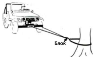
Рис. 20.7 Использование блока дает механическое усилие 2:1. К тому же вдвое уменьшается нагрузка на трос и лебедку. Соответственно, мотор будет крутить быстрее и с меньшим потреблением энергии. Можно работать с длинным тросом и не бояться перегрева мотора
