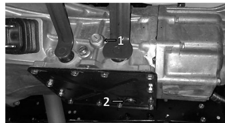
Рис. 9.1 Коробка передач HYUNDAI DYMOS M5ZR1:
