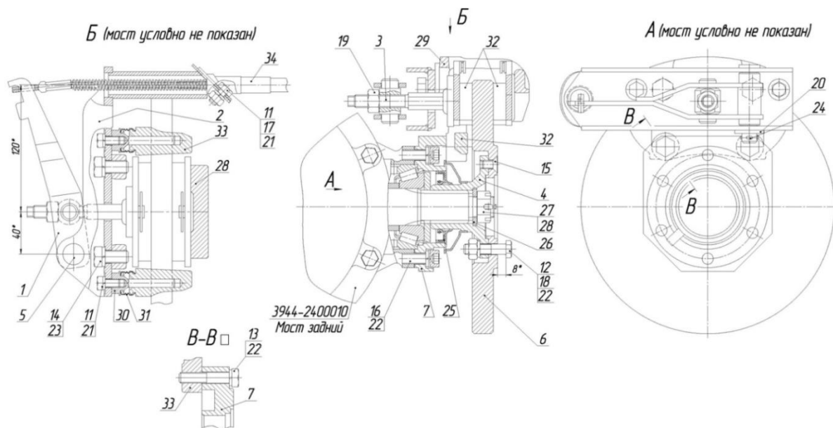
Рис. 6.18 Устройство стояночного тормоза
