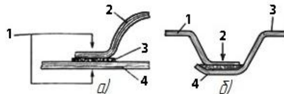
Рис. 6.22. Соединение слоистого пластика склеиванием:
