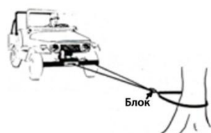
Рис. 20.2 Использование блока дает механическое усилие 2:1. К тому же вдвое уменьшается нагрузка на трос и лебедку. Соответственно, мотор будет крутить быстрее и с меньшим потреблением энергии. Можно работать с длинным тросом и не бояться перегрева мотора
