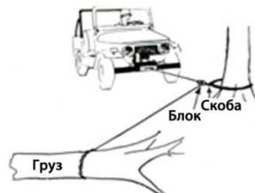
Рис. 20.4 Пример того, как с помощью блока можно менять направление тяги. Блок подсоединяется к древозащитной ленте с помощью соединительной скобы
