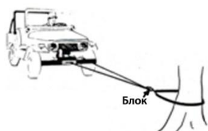
Рис. 20.6 Использование блока дает механическое усилие 2:1. К тому же вдвое уменьшается нагрузка на трос и лебедку. Соответственно, мотор будет крутить быстрее и с меньшим потреблением энергии. Можно работать с длинным тросом и не бояться перегрева мотора
