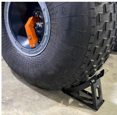
Рис.20.36 Упор противооткатный
