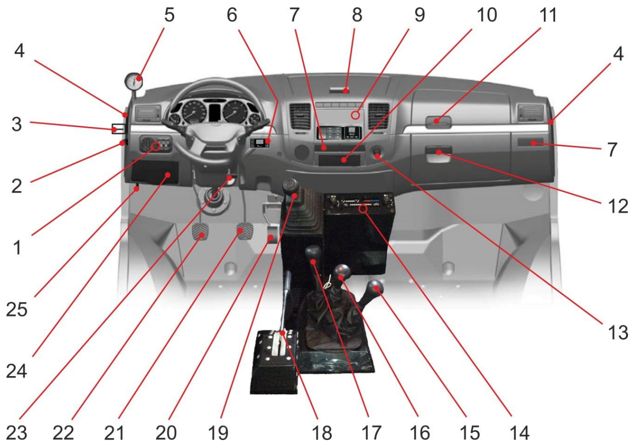
Рис. 5.6 Органы управления:
