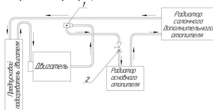
Рис. 6.20. Система отопления:
