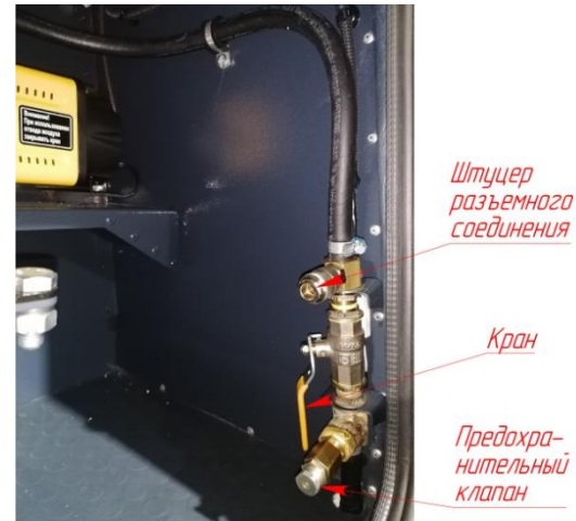
Рис. 20.1 Узел отвода воздуха
