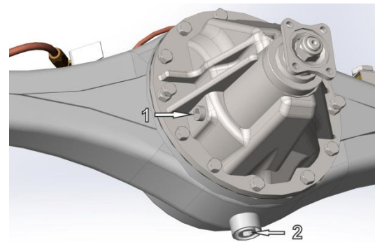
Рис. 9.5 Картер главной передачи ведущего моста:
