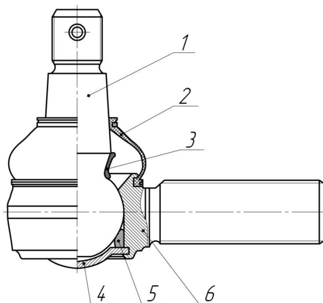
Рис. 6.16 Нерегулируемый наконечник рулевой тяги
