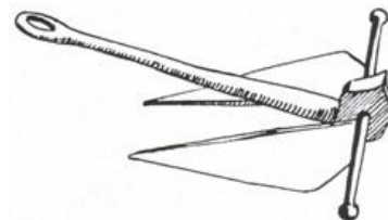
Рис. 19.9 Специальный якорь. В качестве такового лучше всего подходит лодочный якорь. Десятикилограммового якоря достаточно практически в любой почве и легко вытаскивается – достаточно проехать над ним. Для большей эффективности неплохо свести якоря вдвое ближе к стержню
