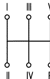
Рис. 6.1 Схема управления коробками передач
