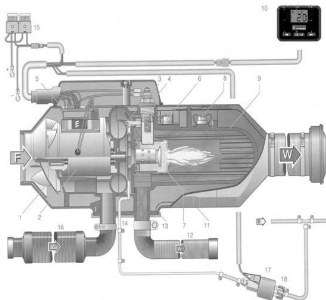
Рис. 19.12 AIRTRONIC B4 в разрезе (Бензин)
