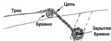
Рис. 19.8 Зарытое в землю бревно – отличный якорь. При необходимости вместо бревна можно использовать целый ряд предметов, например, металлическую балку, трубу или даже большую канистру.
