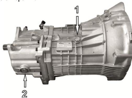
Рис. 9.2 Коробка передач HYUNDAI T032S5: 1 - пробка заливного (контрольного) отверстия, 2 - пробка сливного отверстия.
