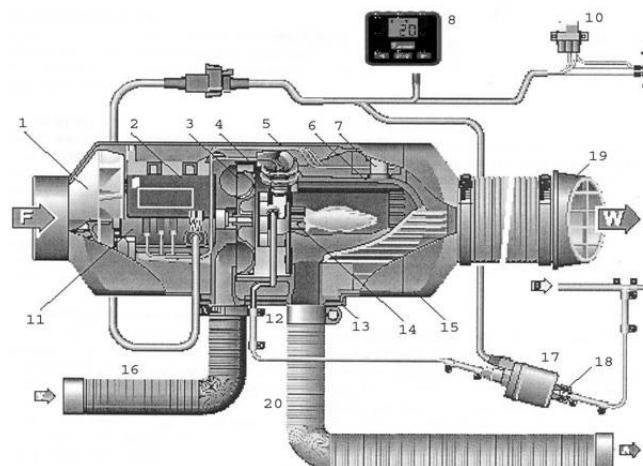
Рис. 19.11 AIRTRONIC D4 в разрезе (Дизель):
