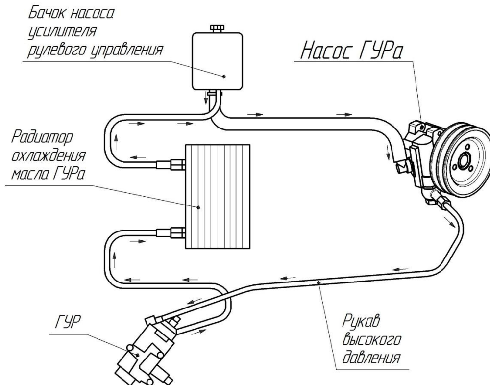
Рис. 6.13 Общая схема гидросистемы рулевого управления
