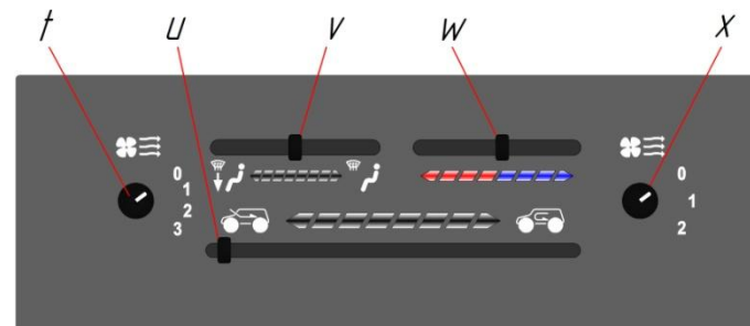
Рис. 5.11 Блок управления отопителем
