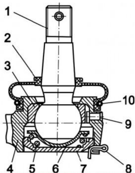
Рис. 6.15 Регулируемый наконечник рулевой тяги
