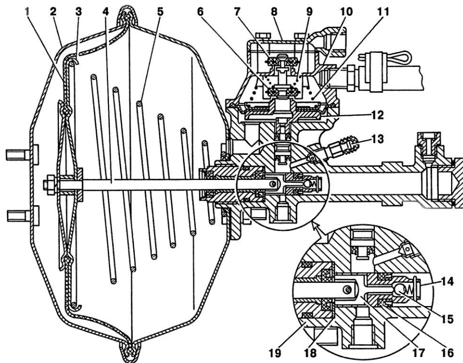
Рис. 6.19 Гидровакуумный усилитель
