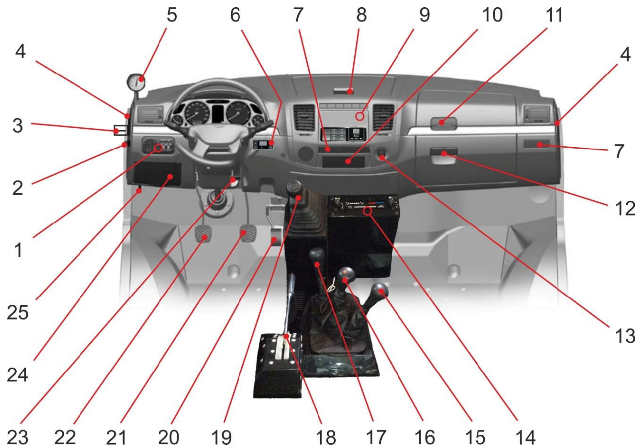
Рис. 5.6 Органы управления:
