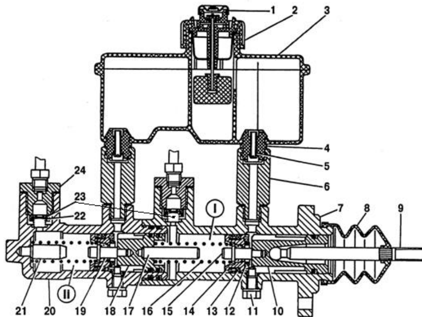
Рис.6.16 Главный тормозной цилиндр
