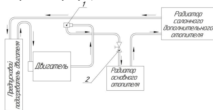
Рис. 6.20. Система отопления:
