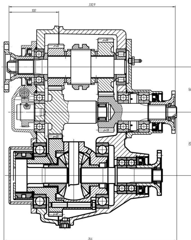
Рис.6.4 Коробка привода заднего ведущего моста с приводом водомётного движителя
