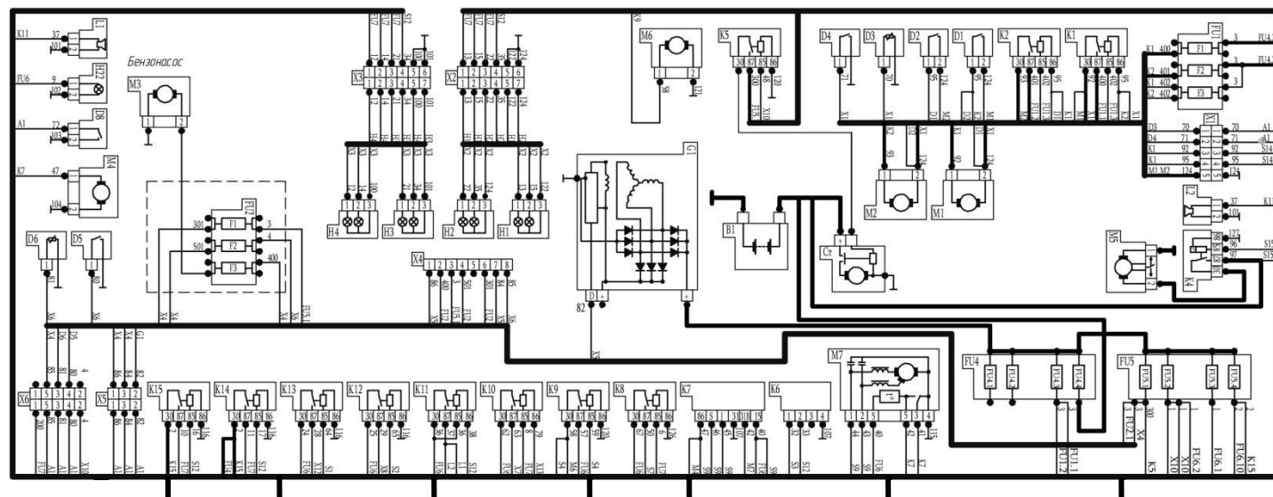
Рис 6.19 (Часть 1) Базовая электрическая схема ВТС
