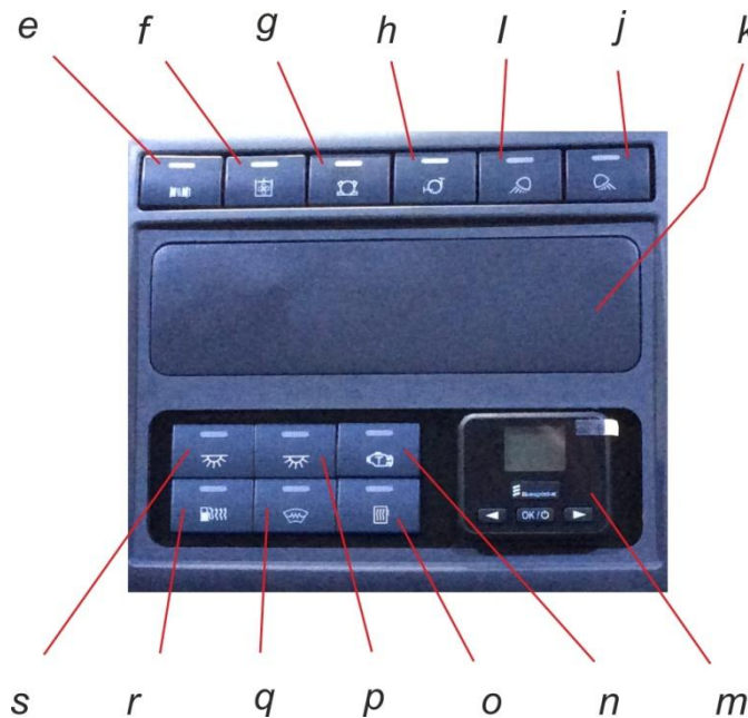
Рис. 5.8 Центральная панель
