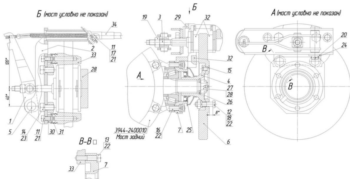
Рис. 6.18 Устройство стояночного тормоза
