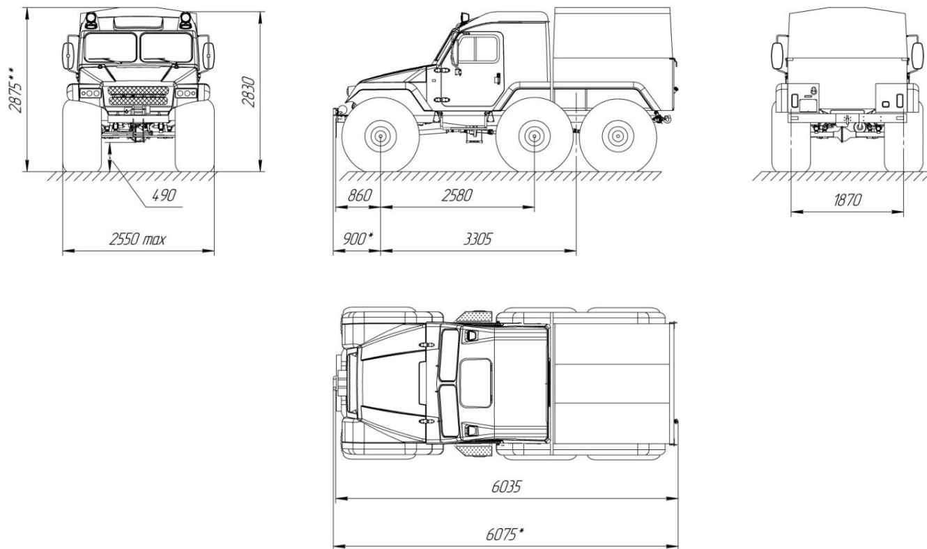
Рис. 5.2 Основные размеры ВТС ТРЭКОЛ 39295
