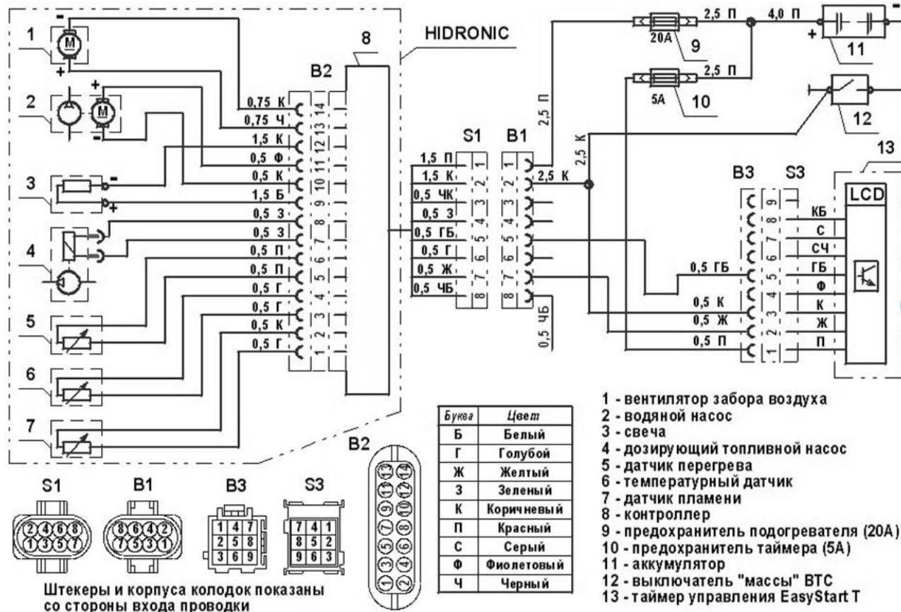
Рис. 20.15 Электрическая схема подключения подогревателя
