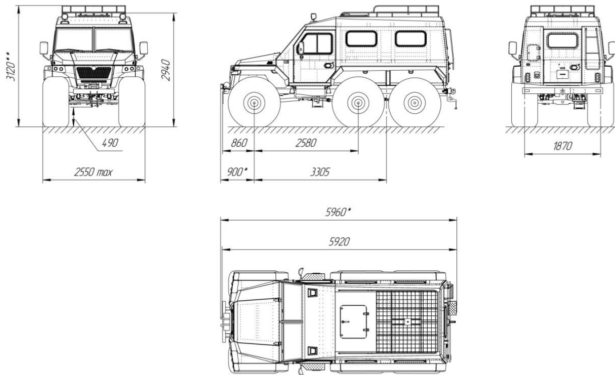
Рис. 5.3 Основные размеры ВТС ТРЭКОЛ ВЕГА
