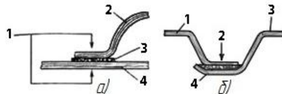
Рис. 6.22. Соединение слоистого пластика склеиванием:
