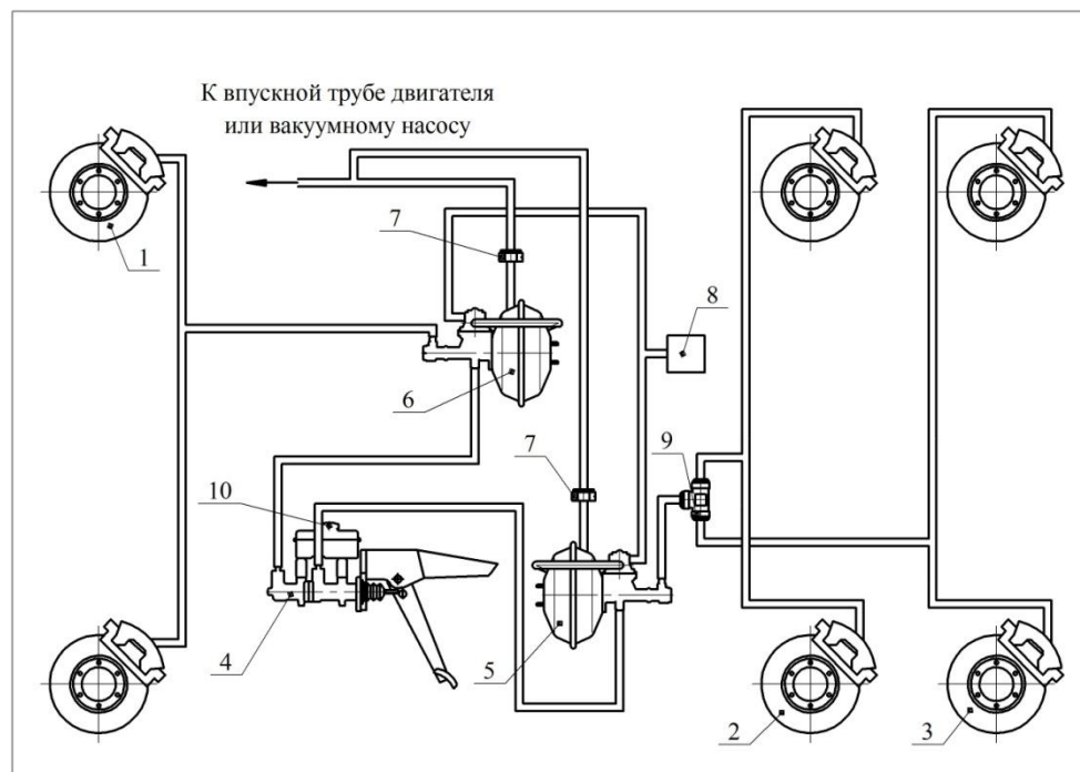
Рис. 6.15 Схема гидропривода тормозов:
