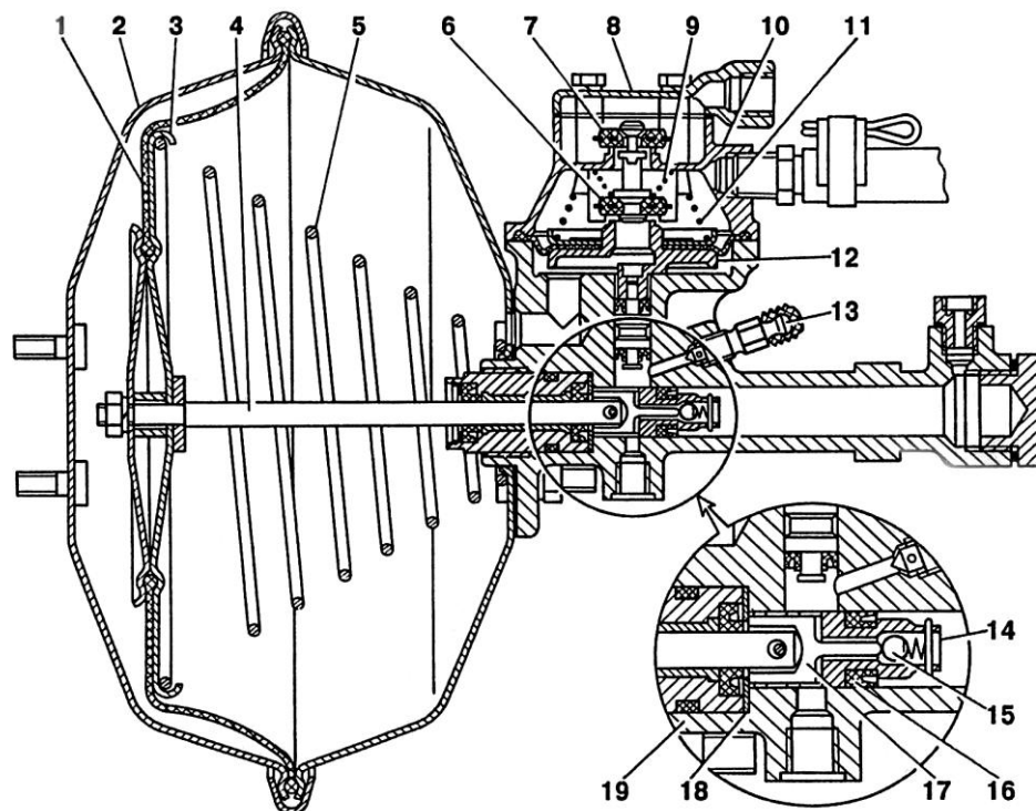
Рис. 6.17 Гидровакуумный усилитель
