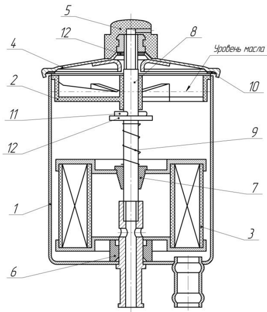
Рис. 6.14 Бачок усилителя рулевого управления: 1 – корпус; 2 - фильтр заливной; 3 – элемент фильтрующий; 4 –крышка; 5 - пробка; 6 – вставка; 7 – шайба фильтра; 8 – шпилька; 9 – пружина клапана; 10 - прокладка уплотнительная; 11 – шплинт; 12 – шайба.
