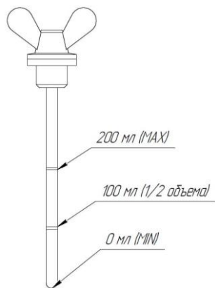
Рисунок 20.3. Указатель уровня антифриза
