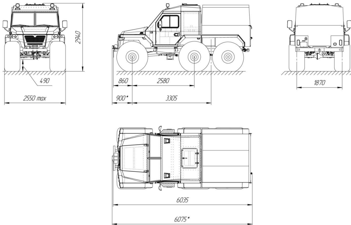
Рис. 5.4 Основные размеры ВТС ТРЭКОЛ ВЕГА Пикап
