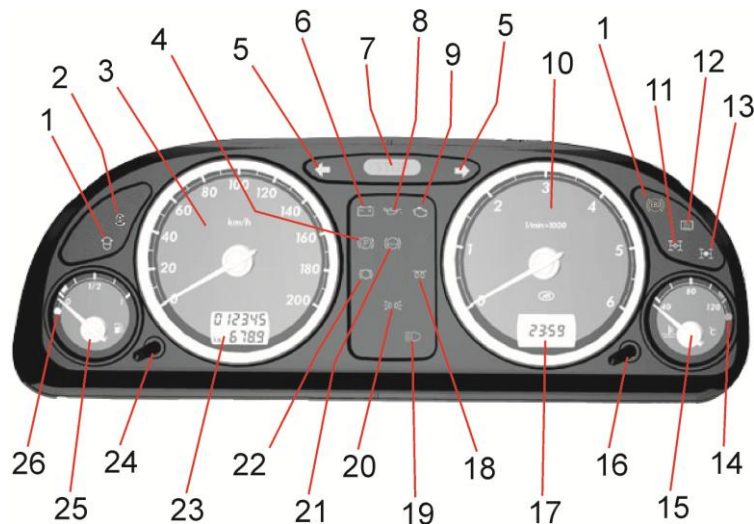
Рис. 5.5 Приборы:
