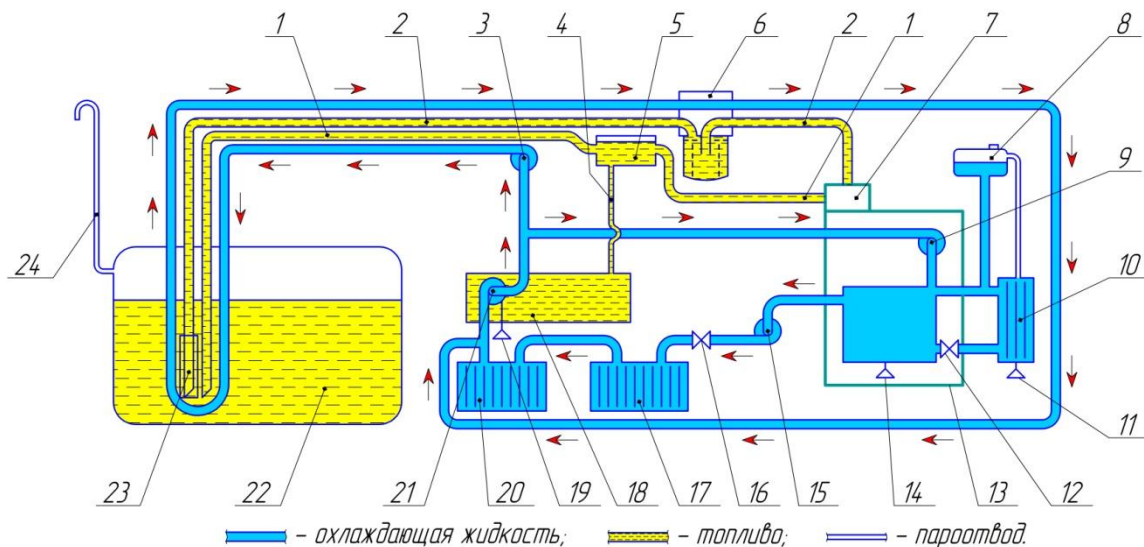
Рис. 20.21 Схема работы системы жидкостного подогрева топливной магистрали
