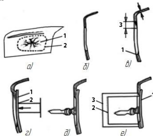
Рис. 6.21. Заделка сквозного повреждения:
