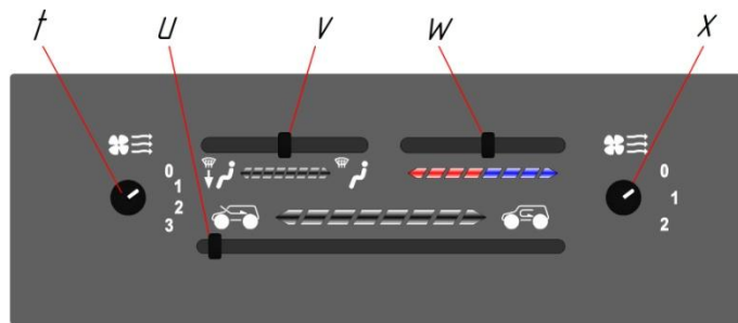
Рис. 5.9 Блок управления отопителем
