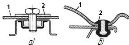
Рис. 6.23. Соединение слоистый пластик-слоистый пластик:
