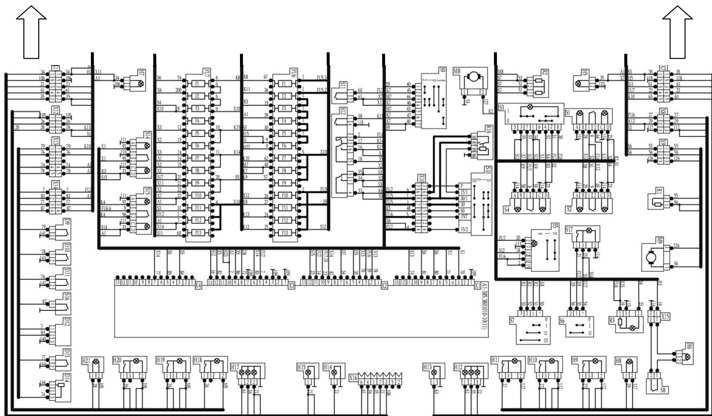
Рис 6.19 (Часть 2) Базовая электрическая схема ВТС
