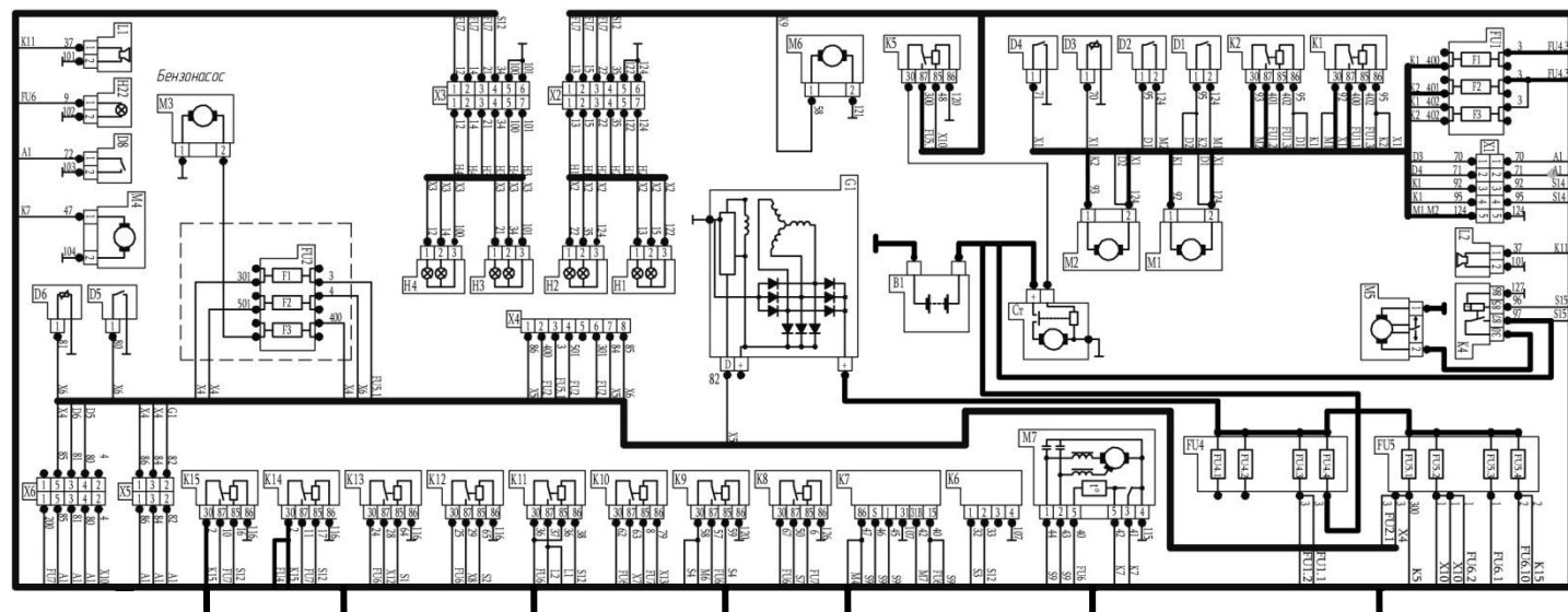
Рис 6.19 (Часть 1) Базовая электрическая схема ВТС
