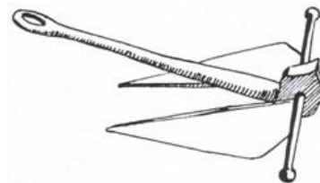
Рис. 20.9 Специальный якорь. В качестве такового лучше всего подходит лодочный якорь. Десятикилограммового якоря достаточно практически в любой почве и легко вытаскивается – достаточно проехать над ним. Для большей эффективности неплохо свести якоря вдвое ближе к стержню
