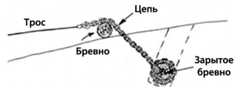
Рис. 20.8 Зарытое в землю бревно – отличный якорь. При необходимости вместо бревна можно использовать целый ряд предметов, например, металлическую балку, трубу или даже большую канистру.
