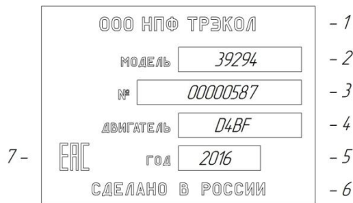
Рис. 4.2 Идентификационная табличка ВТС:
