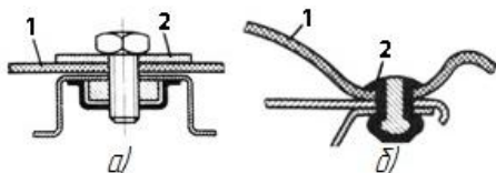
Рис. 6.22. Соединение слоистый пластик-слоистый пластик:
