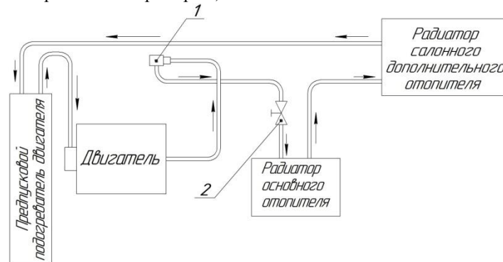
Рис. 6.19. Система отопления:
