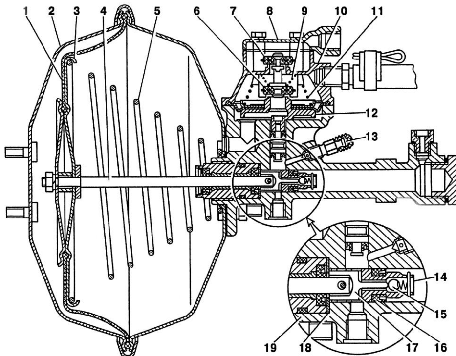
Рис. 6.16 Гидровакуумный усилитель
