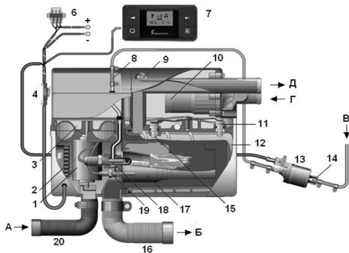
Рис. 20.17 HYDRONIC В 4 W SC и В 5 W SC в разрезе (бензин):
