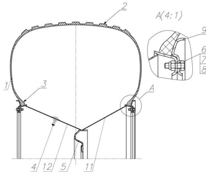
Рис. 10.1 Шина 1300х600-533 ТРЭКОЛ с колесом в сборе
