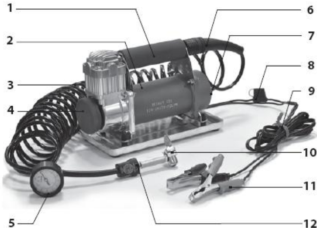
Рис. 12.2 Компрессор:
