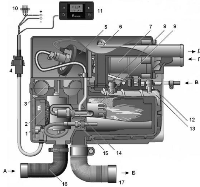
Рис. 20.16 HYDRONIC D 4 W SC и D5 W SC в разрезе (дизель)
