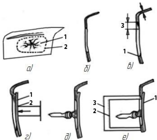
Рис. 6.20. Заделка сквозного повреждения:
