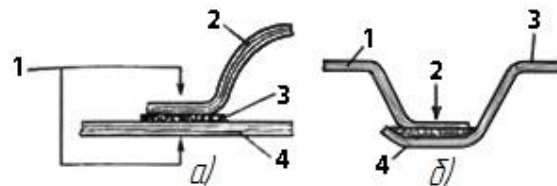
Рис. 6.21. Соединение слоистого пластика склеиванием:
