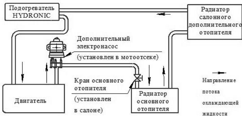
Рис. 20.18 Схема подключения подогревателя к системе охлаждения двигателя
