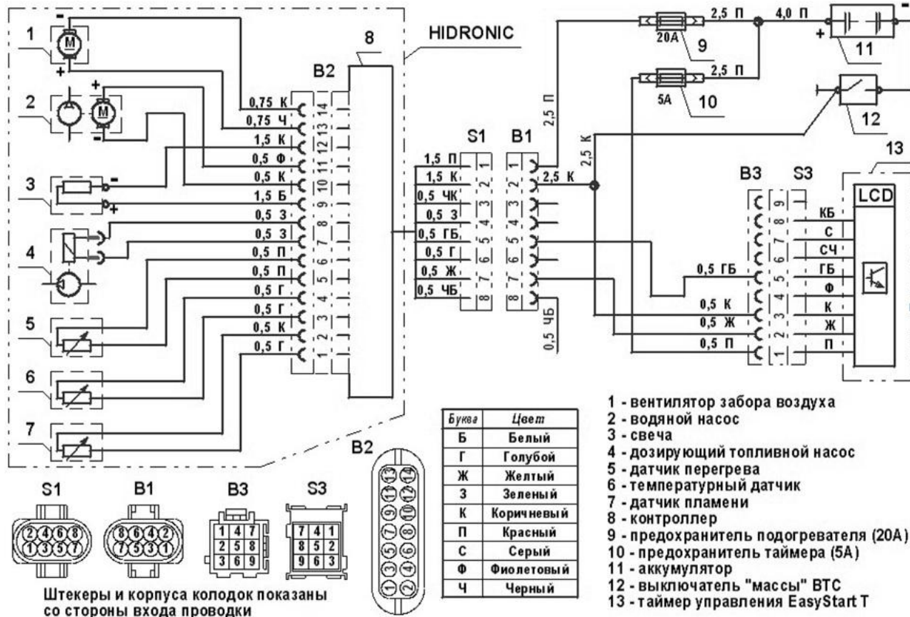
Рис. 20.19 Электрическая схема подключения подогревателя
