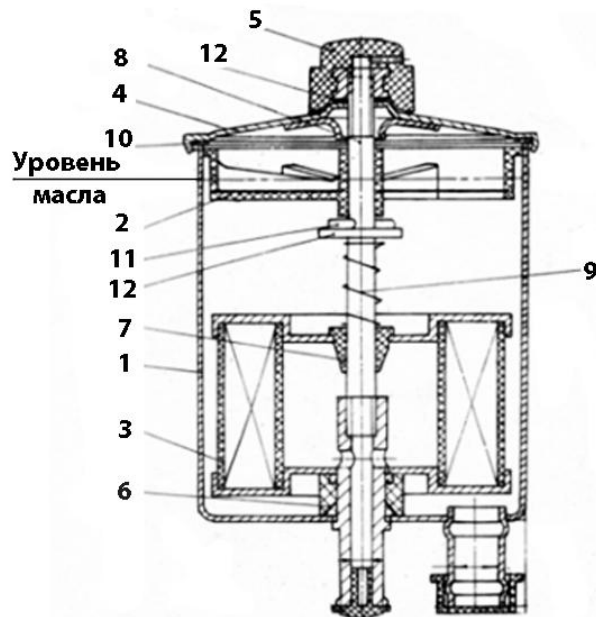
Рис. 6.13 Бачок усилителя рулевого управления: 1 – корпус; 2 - фильтр заливной; 3 – элемент фильтрующий; 4 – крышка; 5 - пробка; 6 – вставка; 7 – шайба фильтра; 8 – шпилька; 9 – пружина клапана; 10 - прокладка уплотнительная; 11 – шплинт; 12 – шайба.
