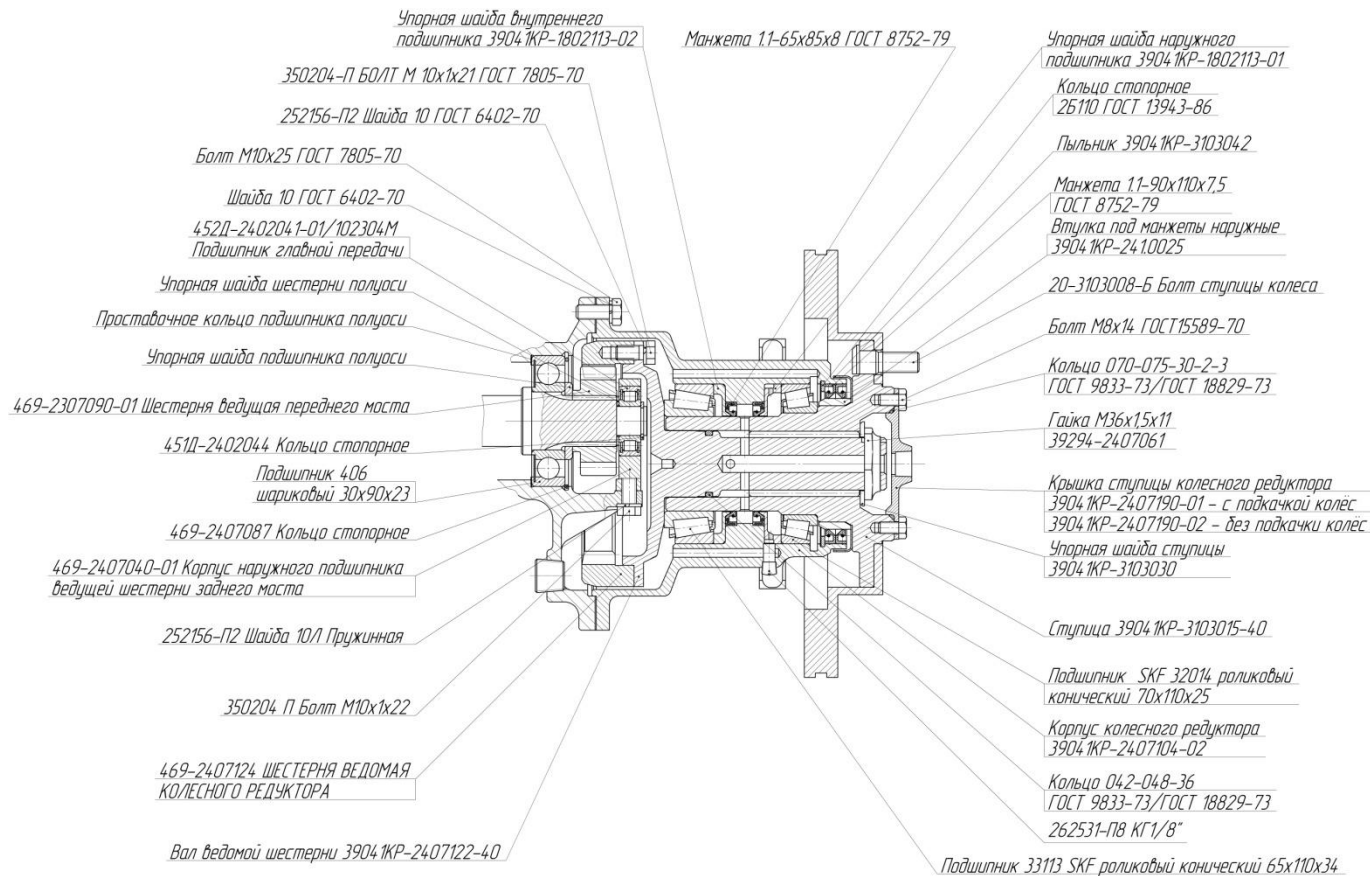
Рис. 6.11 Редуктор ТРЭКОЛ
