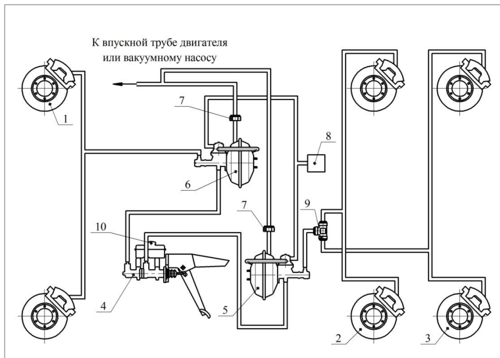
Рис. 6.14 Схема гидропривода тормозов:
