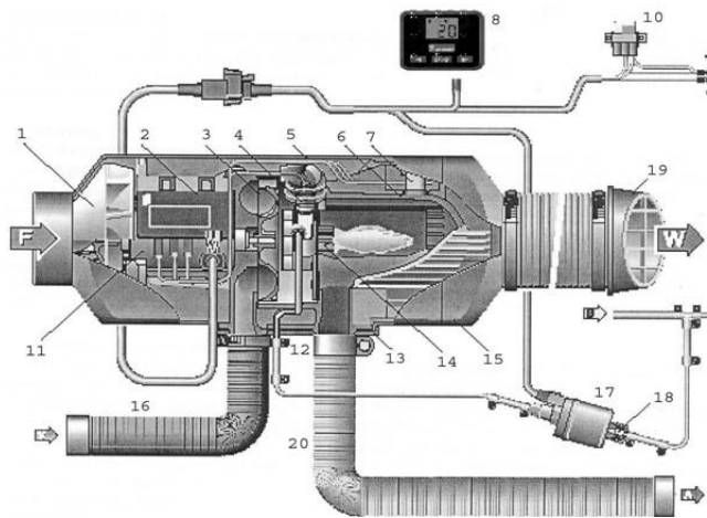
Рис. 20.20 AIRTRONIC D4 в разрезе (Дизель):
