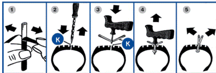
Рис.10.3 Ремонт шины ТРЭКОЛ шнуром (без демонтажа)
