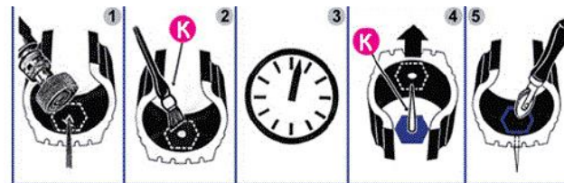
Рис.10.5 Ремонт шины ТРЭКОЛ грибком (с демонтажем)
