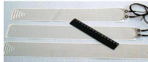
Рис.20.35 Подогрев ветрового стекла
