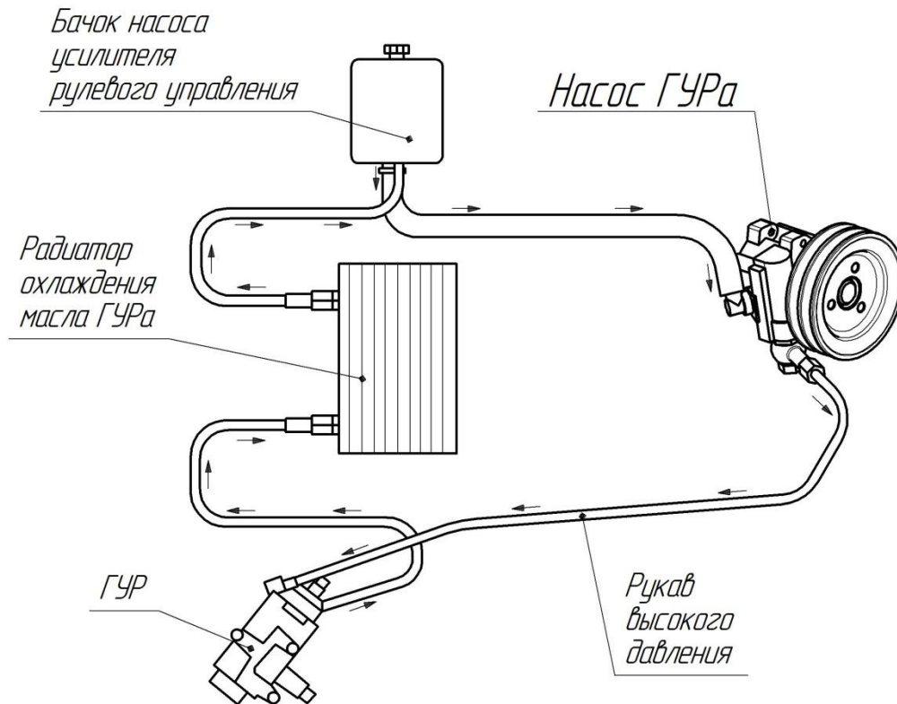
Рис. 6.12 Общая схема гидросистемы рулевого управления
