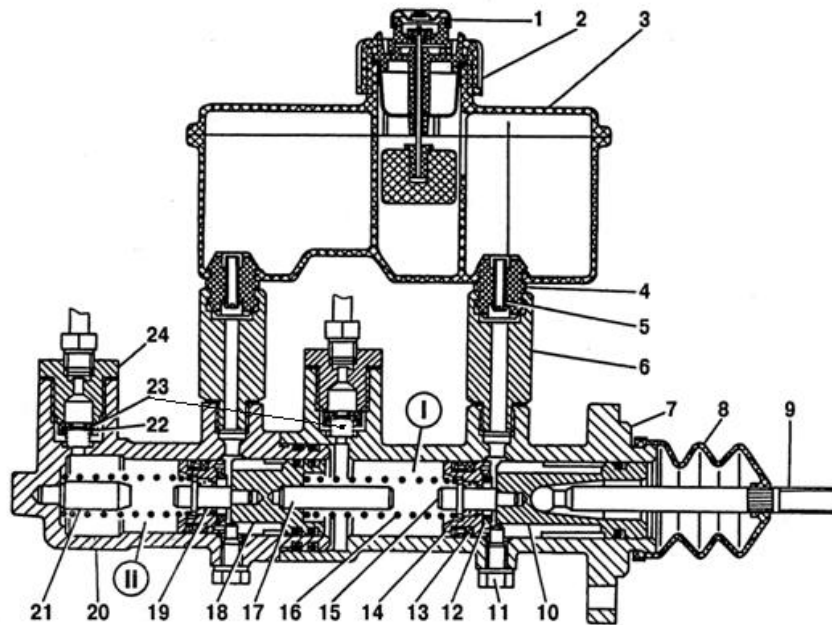
Рис.6.15 Главный тормозной цилиндр
