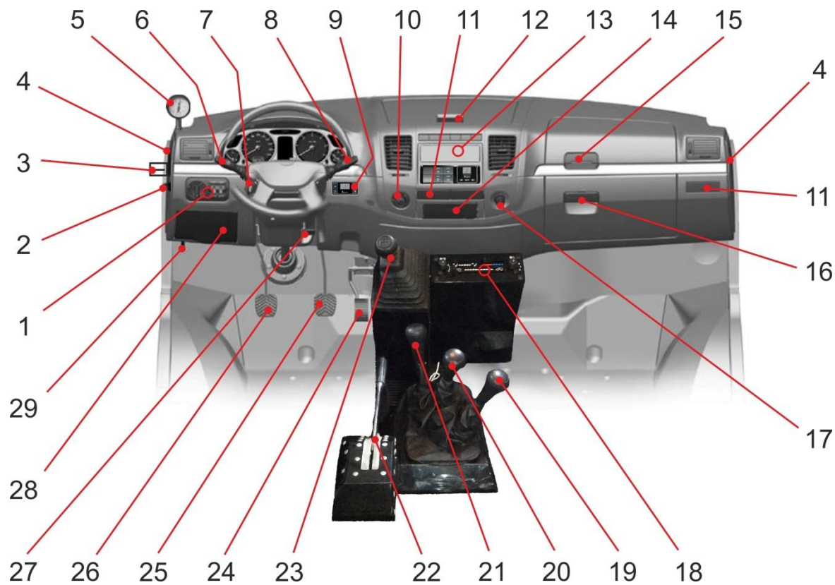
Рис. 5.3 Органы управления:
