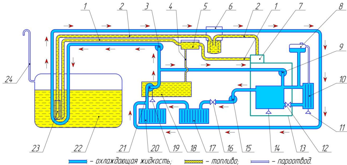
Рис. 20.27 Схема работы системы жидкостного подогрева топливной магистрали
