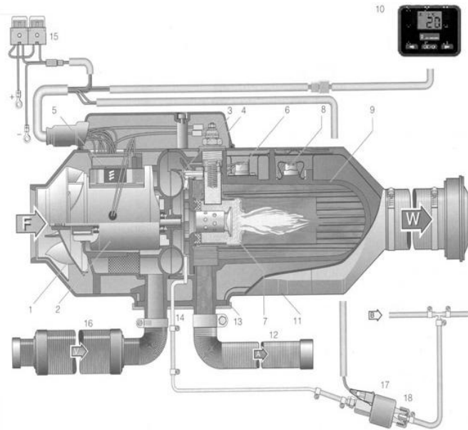
Рис. 20.21 AIRTRONIC B4 в разрезе (Бензин)
