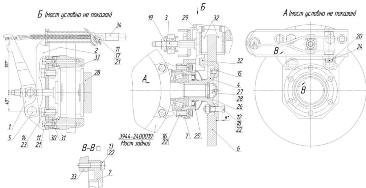
Рис. 6.17 Устройство стояночного тормоза
