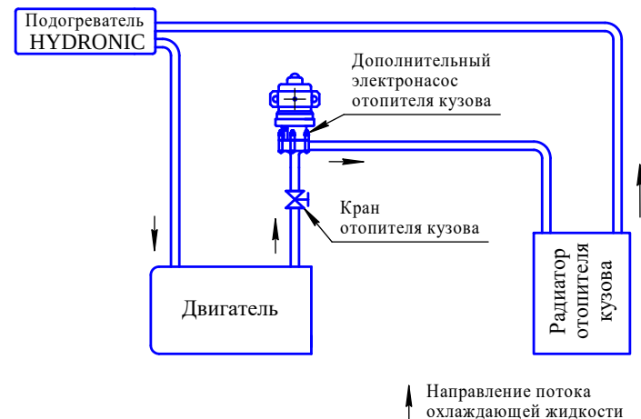
Рис. 20.11 Схема подключения подогревателя к системе охлаждения двигателя
