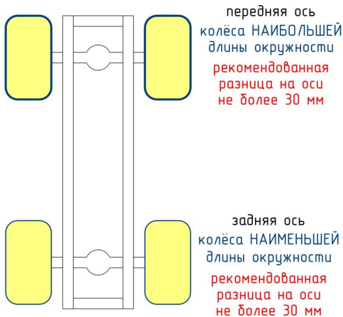
Рис. 10.1 Расстановка колёс
