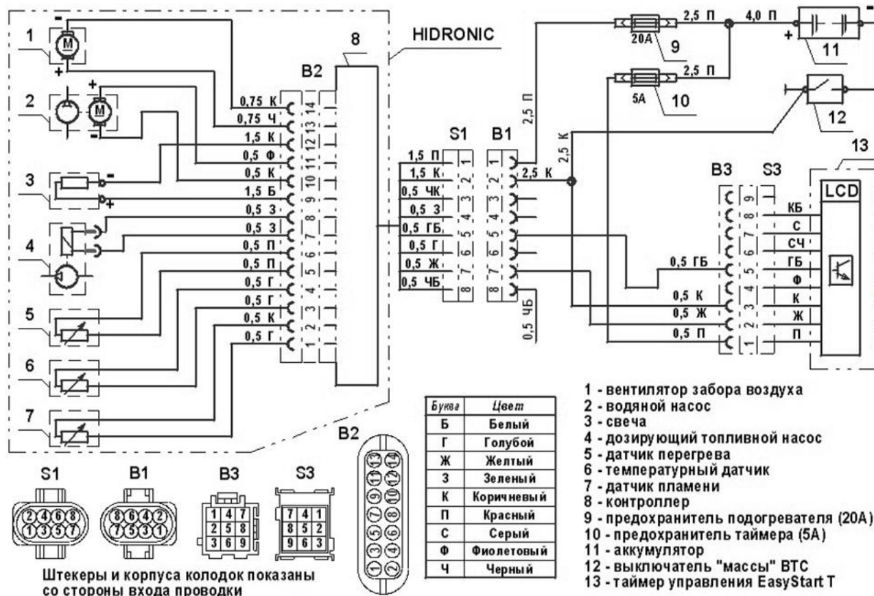
Рис. 20.12 Электрическая схема подключения подогревателя
