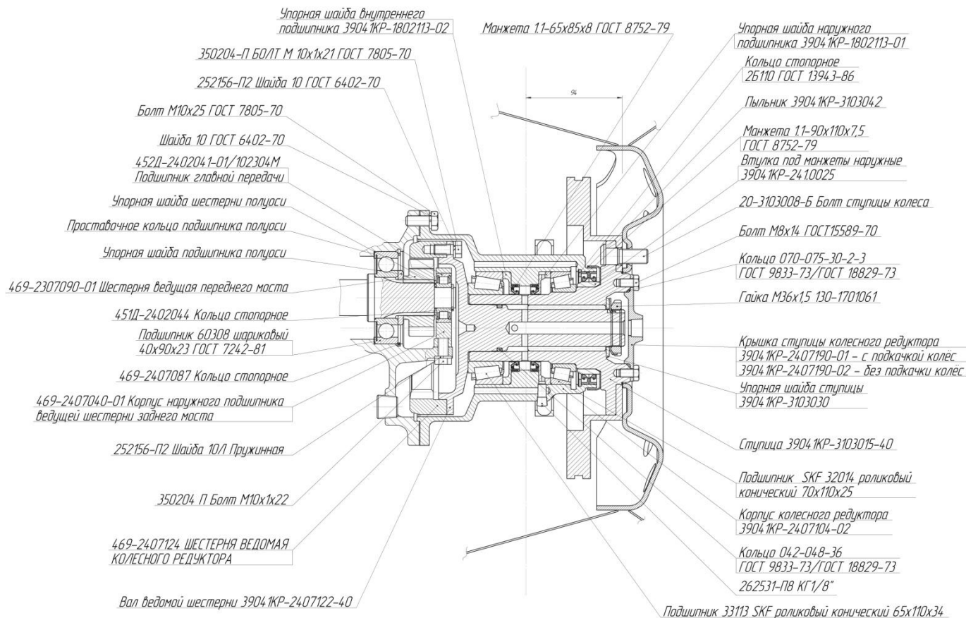
Рис. 6.3 Редуктор ТРЭКОЛ-39041К
