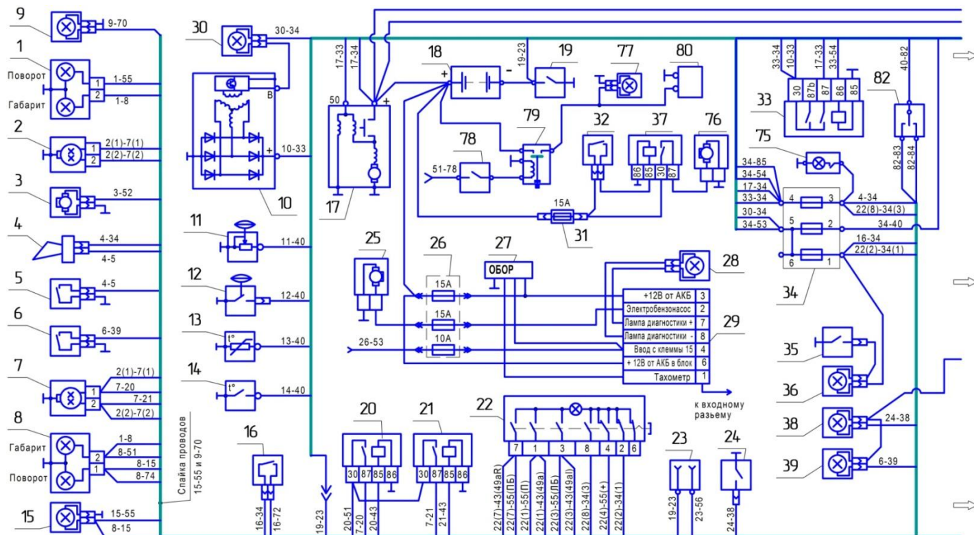
Рис. 6.7 (часть 1) Базовая электрическая схема ВТС
