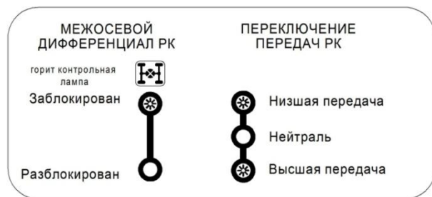
Рис. 6.2 Схема управления раздаточной коробкой
