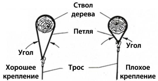
Рис. 20.7 Петля.
