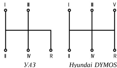
Рис. 6.1 Схемы переключения коробок передач УАЗ и Hyundai DYMOS
