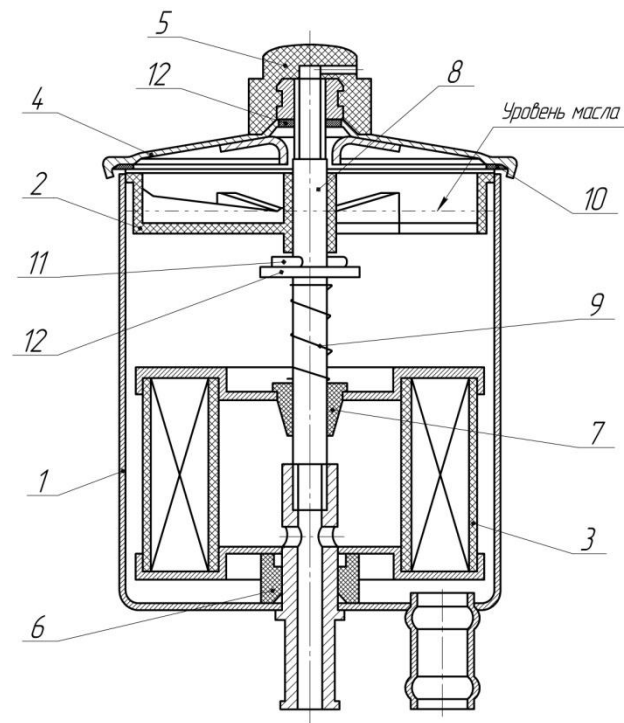
Рис. 6.5 Бачок усилителя рулевого управления:
