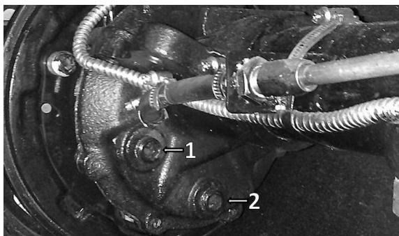
Рис. 9.6 Картер бортовой передачи: 1 - пробка заливного (контрольного) отверстия, 2 - пробка сливного отверстия
