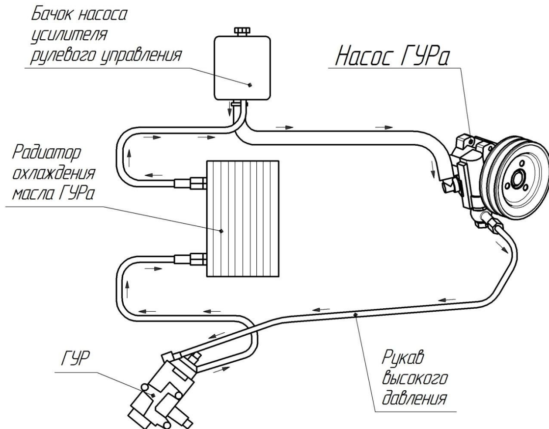
Рис. 6.4 Общая схема гидросистемы рулевого управления
