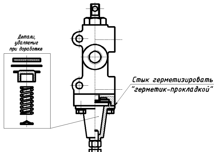
Рис. 20.1. Доработка крана управления.
