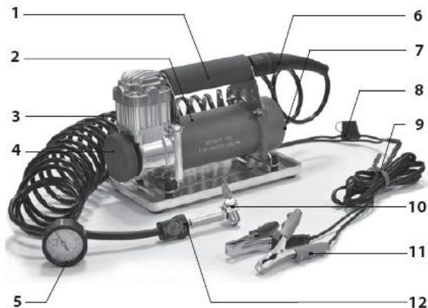
Рис. 12.2 Компрессор:
