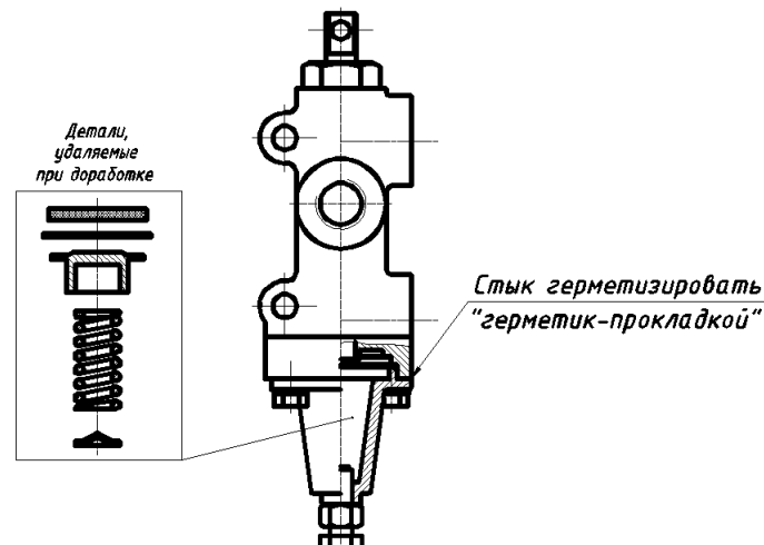
Рис. 20.5. Доработка крана управления 11.3122009-02.
