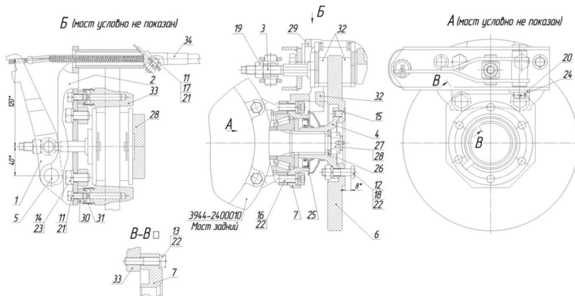
Рис. 6.6 Устройство стояночного тормоза
