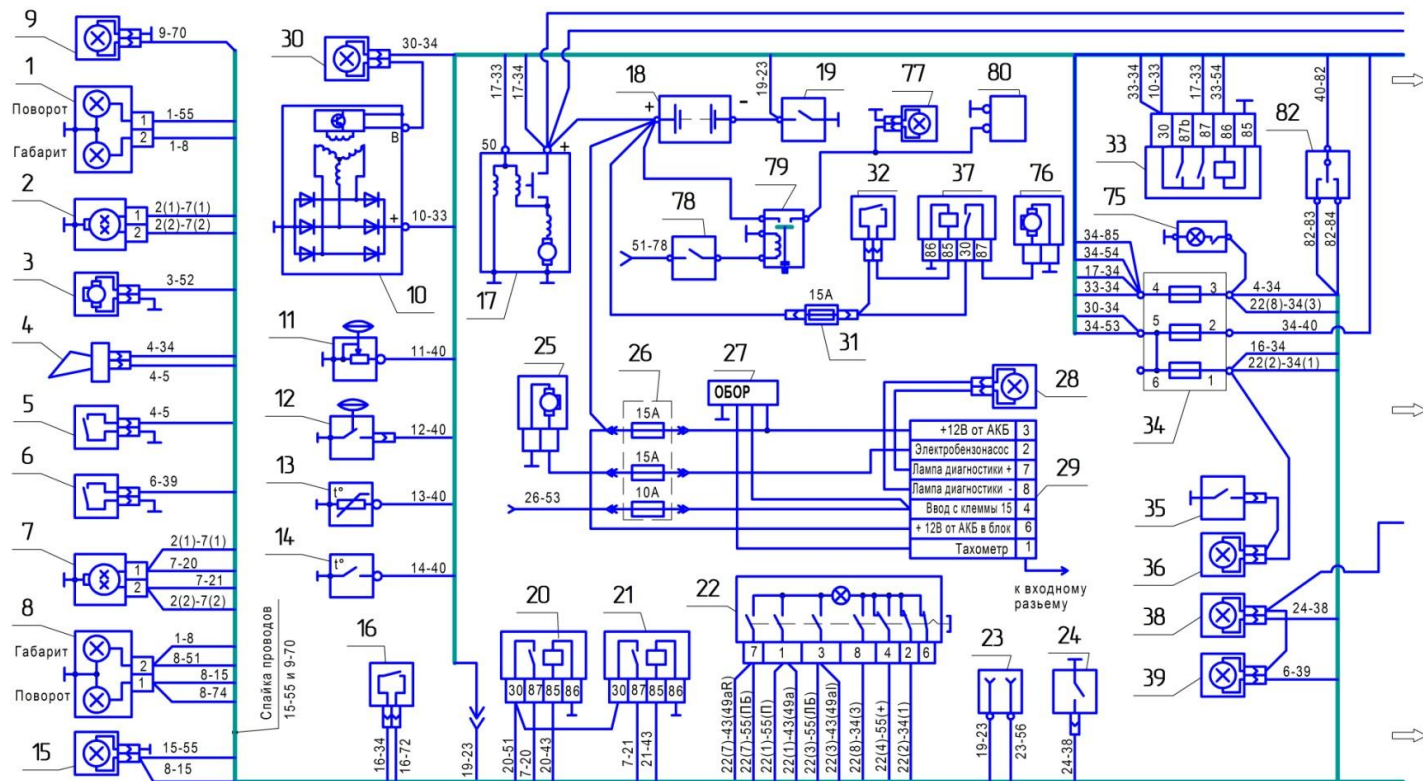
Рис. 6.7 (часть 1) Схема электропитания ТРЭКОЛ 39041
