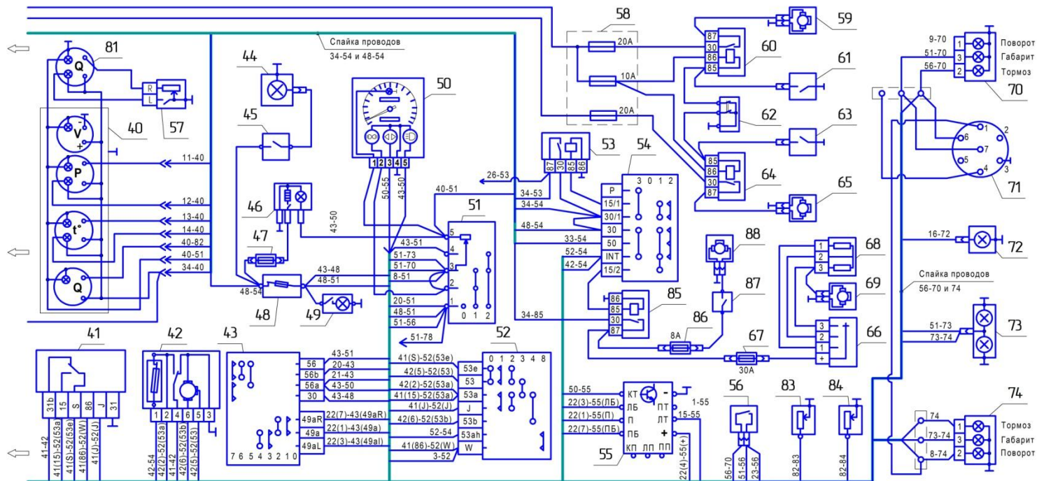
Рис. 6.7 (часть 2) Схема электропитания ТРЖОЛ 39041
